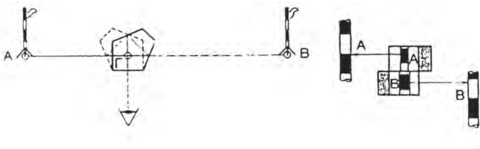
Σχ. 45 Διαδικασία πύκνωσης ευθυγραμμίας με το ορθόγωνο.
