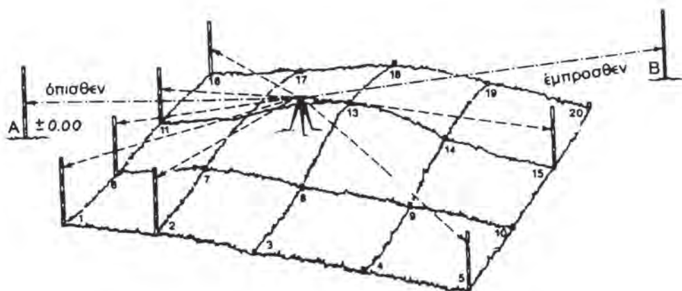
Σχ. 69 Με τη χωροστάθμιση επιφανείας δίνονται υψόμετρα σε όλα τα σημεία του κανάβου.
