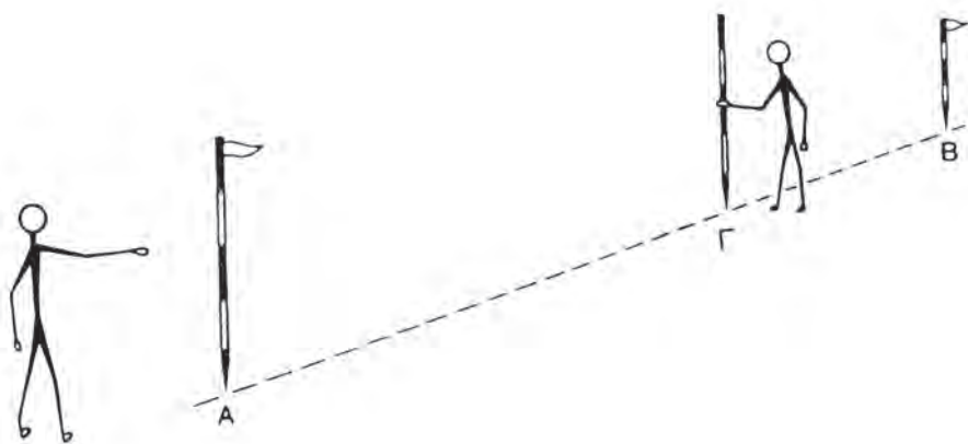
Σχ. 31 Τοποθέτηση του τρίτου ακοντίου στην ευθυγραμμία.
