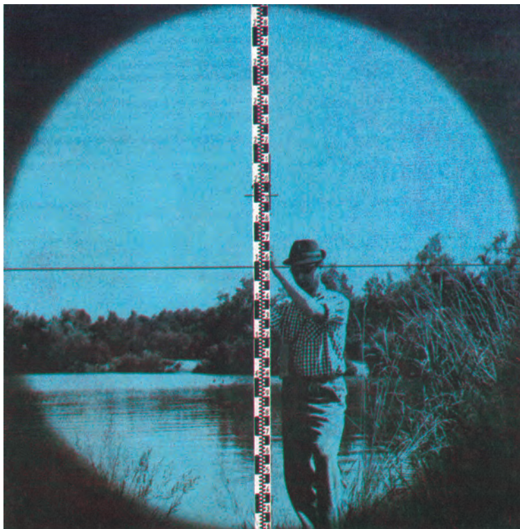
Εικ. 25 Η εικόνα που έχουμε όταν σκοπεύουμε τη σταδία με το χωροβάτη. Το οριζόντιο νήμα του σταυρονήματος τέμνει νοητά τη σταδία στην ένδειξη που πρέπει να διαβάσουμε.
