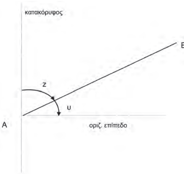
Σχ. 8 Οι κατακόρυφες γωνίες.
