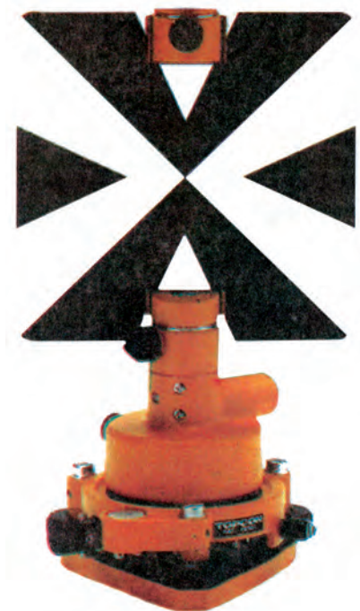
Εικ. 13 Ειδικός στόχος για μετρήσεις γωνιών.
