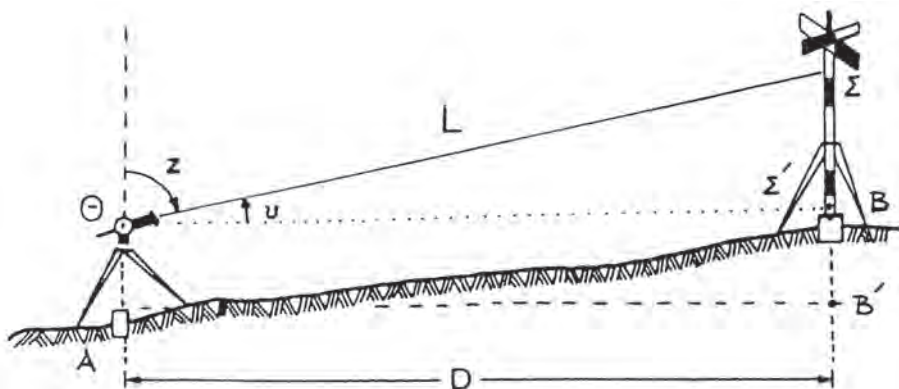
Σχ. 33 Μετριοούνται τα μεγέθη L και z για να υπολογιστεί το D .
