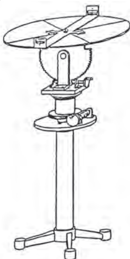
Εικ. 5 Αντίγραφο της διόπτρας του Ήρωνα.
