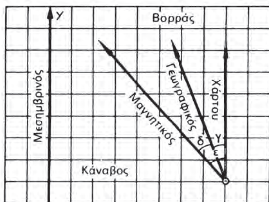
Σχ. 27 Τοπογραφικό διάγραμμα με σχεδιασμένο τον κানাβο και τις διευθύνσεις του γεωγραφικού και του μαγνητικού βορρά.
