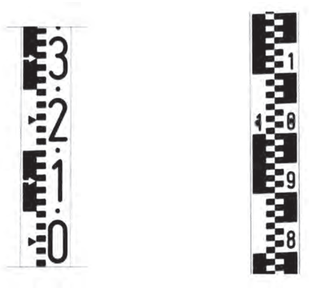
Εικ. 23 Διάφοροι τύποι σταδίων με υποδιαιρέσεις ανά 1cm.
