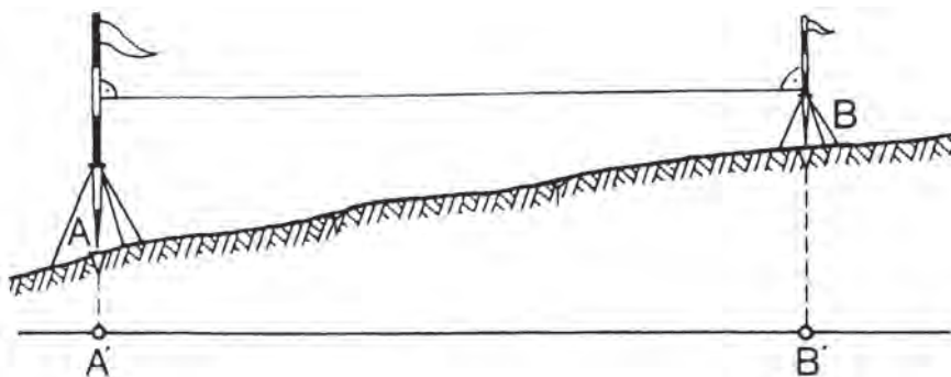
Σχ. 30 Η μετροταινία μετράει την οριζόντια απόσταση A'B' μεταξύ των σημείων A και B.
