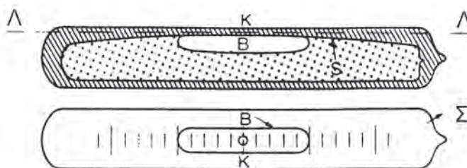
Σχ.22 Τομή και κάτοψη της αεροστάθμης. Το σημείο Κ είναι το κανονικό σημείο.
