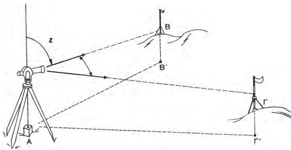
Σχ. 21 Το θεοδόλιχο τοποθετείται στο Α για να μετρήσει οριζόντιες και κατακόρυφες γωνίες
