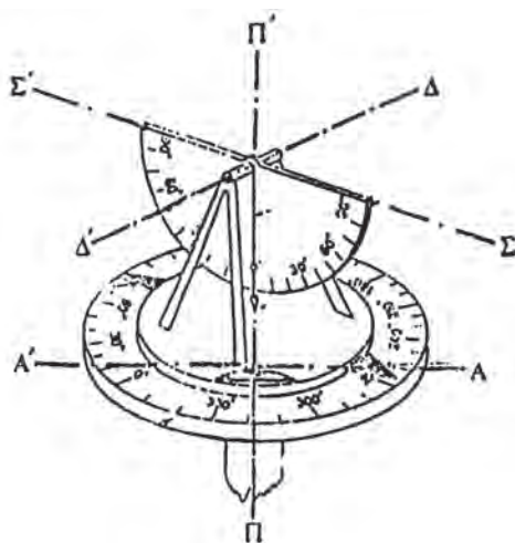
Εικ. 6 Διάταξη που δείχνει ποια είναι η βασική ιδέα λειτουργίας του θεοδολίχου.
