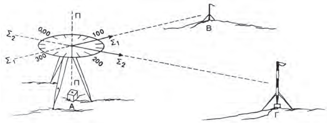
Σχ. 24 Σχηματική παράσταση του οριζόντιου δίσκου του θεοδολίχου και των σκοπευτικών γραμμών προς τα σημεία Β και Γ για τη μέτρηση της οριζόντιας γωνίας.
