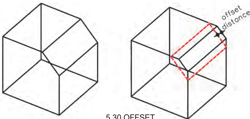
5.30.OFFSET
