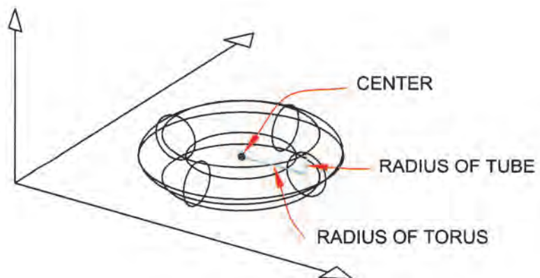
5.11. TORUS
