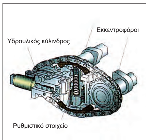
Εικ. 2.4.2 Ρυθμιζόμενος τεντωτήρας αλυσίδας
