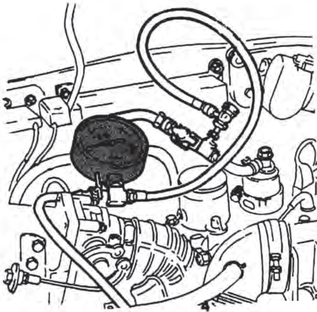
Εικ.3.1.5 Συνδεσμολογία μετρητή πίεσης για τον έλεγχο διατήρησης της πίεσης καυσίμου
