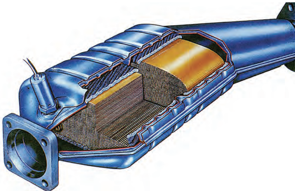
Εικ. 4.4.5 Καταλύτης διπλής κλίνης
