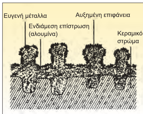
Εικ. 4.4.4 Επίστρωση αλουμίνας
