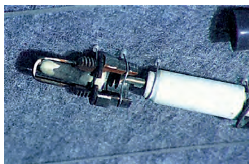
Εικ. 4.5.2 Αισθητήρας «λ»
