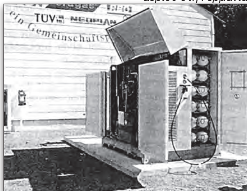
Εικόνα 7.1.11 Σταθμός πλήρωσης φυσικού αερίου στη Γερμανία
