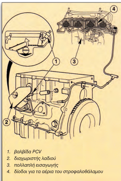
Εικόνα 4.1.13 Εξαερισμός στροφαλο- θάλαμου
