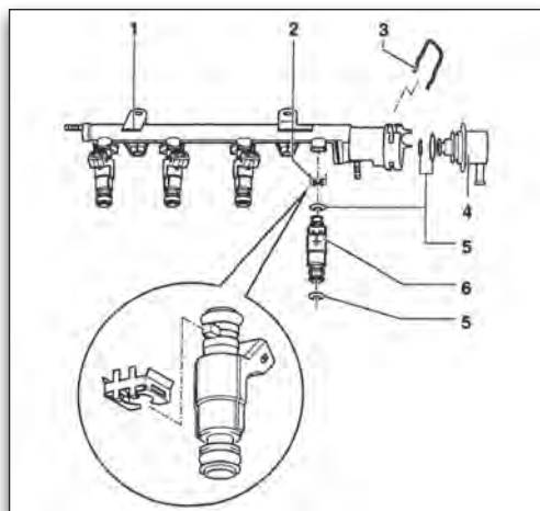
Εικόνα 3.1.13 Διακλαδωτήρας καυσίμου με μπεκ
