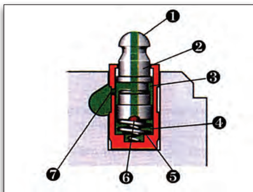
Εικόνα 2.3.2 Υδραυλικό ωστήριο
