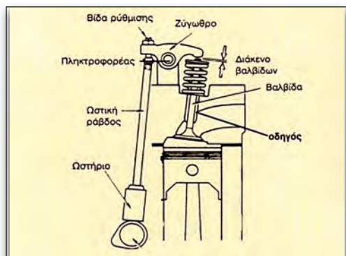
Εικόνα 2.1.6 Βαλβίδα με οδηγό και έδρα
