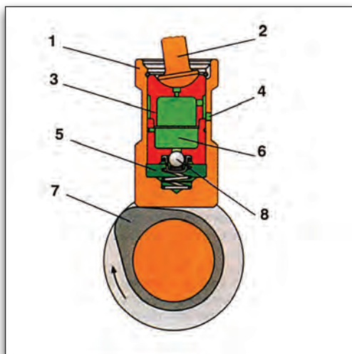
Εικόνα 2.3.3 Λειτουργία ωστηρίου με εκκεντροφόρο επί κεφαλή.
