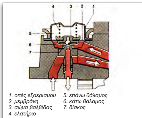
Εικόνα 3.1.23 Μπεκ μονού ψεκασμού με το ρυθμιστή πίεσης
