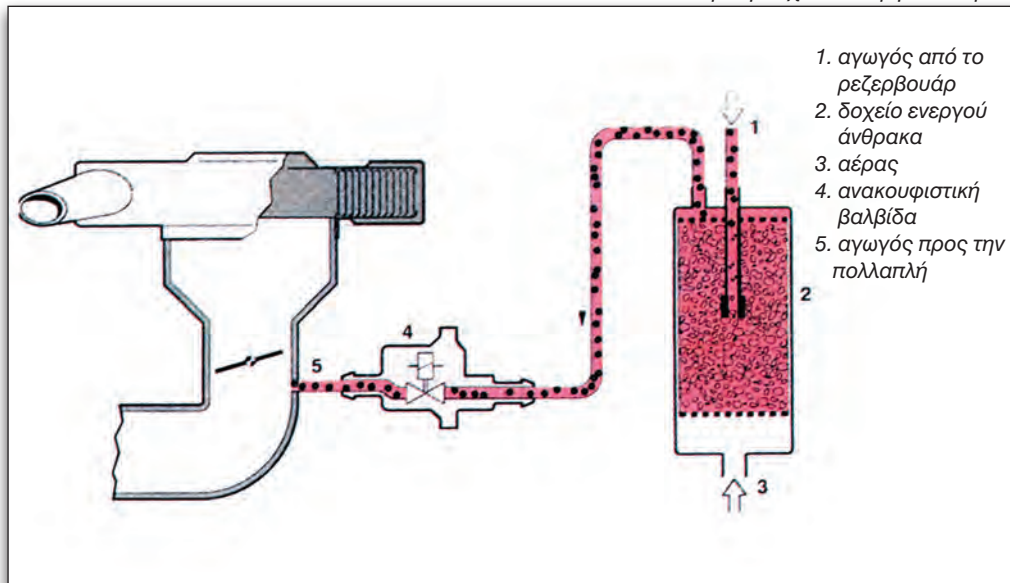
Εικόνα 4.1.3 Ανακούφιση δοχείου ενεργού άνθρακα
