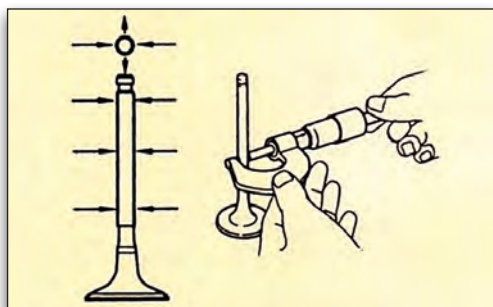
Εικόνα 2.1.9 Μέτρηση βαλβίδας
