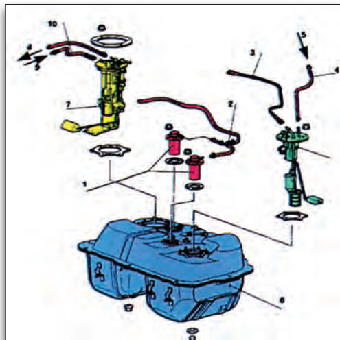
Εικόνα 3.1.7 Συνδεσμολογία ρεζερβουάρ
