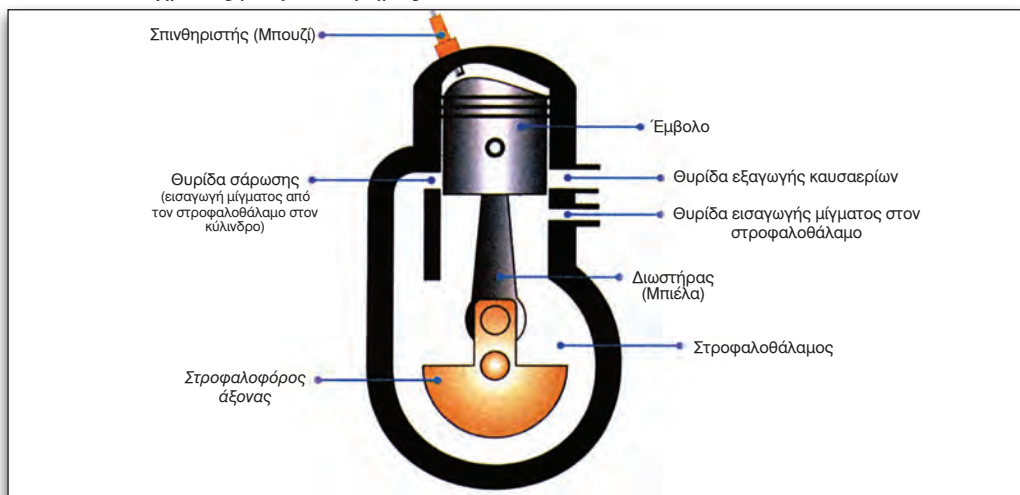
Εικόνα 1.2.9 2χρονος βενζινοκινητήρας
