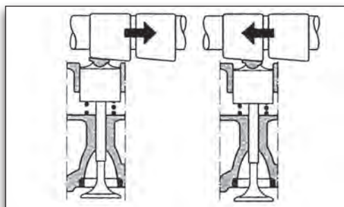
Εικόνα 2.3.10 Συνεχής μεταβολή χρονισμού (FIAT).
