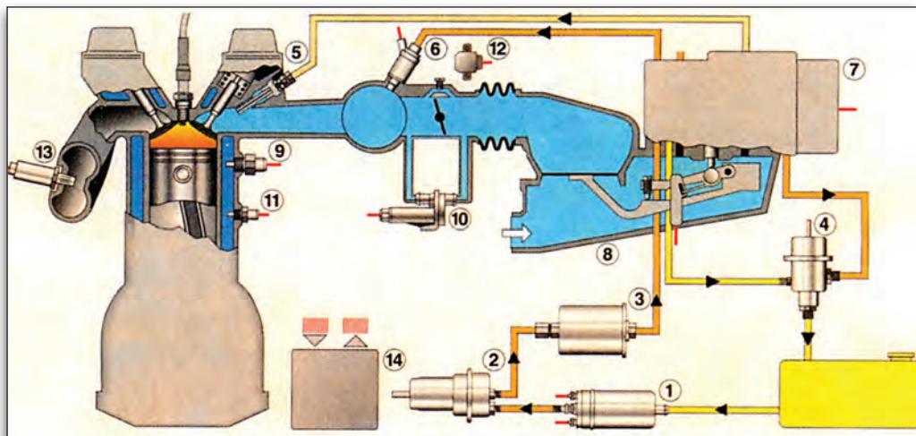
Εικόνα 3.1.46 Σύστημα KE -Jetronic
