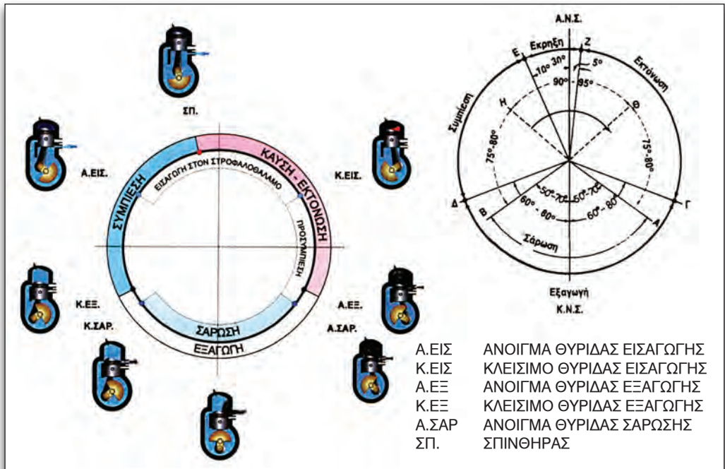
Εικόνα 1.2.11 Κυκλικό διάγραμμα πραγματικής λειτουργίας δίκρονου βενζινοκινητήρα
