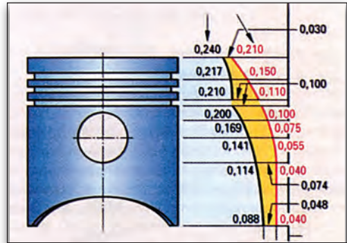
Εικόνα 2.2.5 Κατασκευαστικές λεπτομέρειες εμβόλου
