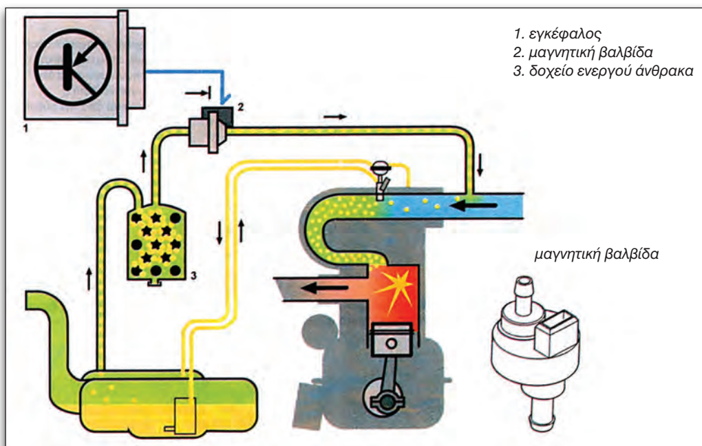
Εικόνα 4.1.4 Εξαερισμός ρεζερβουάρ
