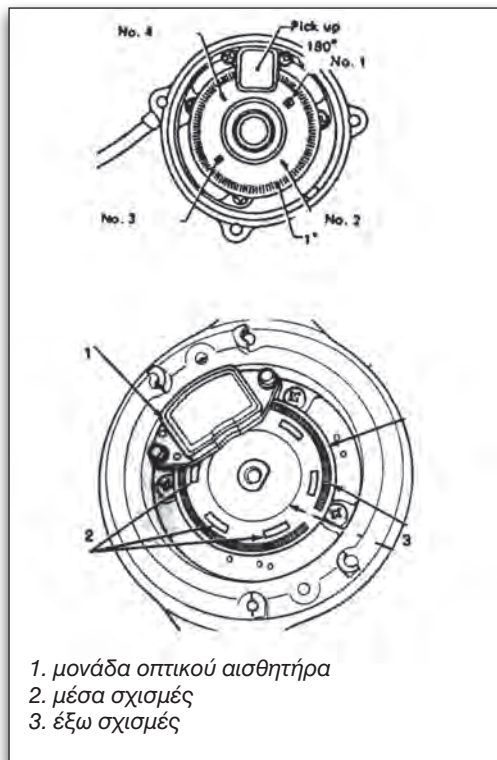
Εικόνα 3.2.17 Σχισμές θέσης εμβόλων τετρακύλινδρου (πάνω) και εξακύλινδρου κινητήρα
