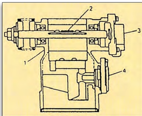
Εικόνα 3.1.31 Σώμα πεταλούδας
