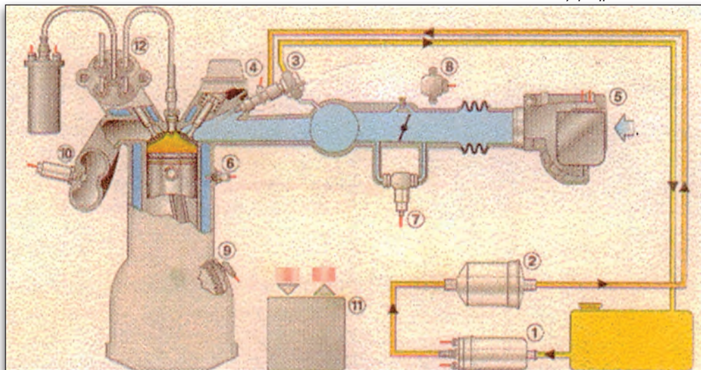
Εικόνα 3.3.4 Εξαρτήματα Motronic
