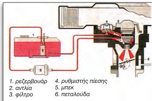
Εικόνα 3.1.22 Ρυθμιστής πίεσης
