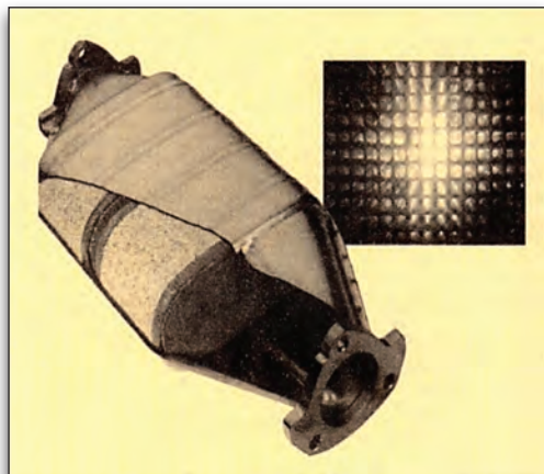
Εικόνα 4.2.5 Τριοδικός καταλύτης
