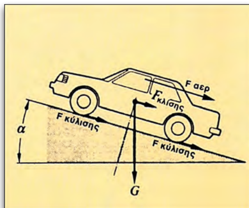
Εικόνα 8.2.6. Οι αντιστάσεις κίνησης ενός αυτοκινήτου
