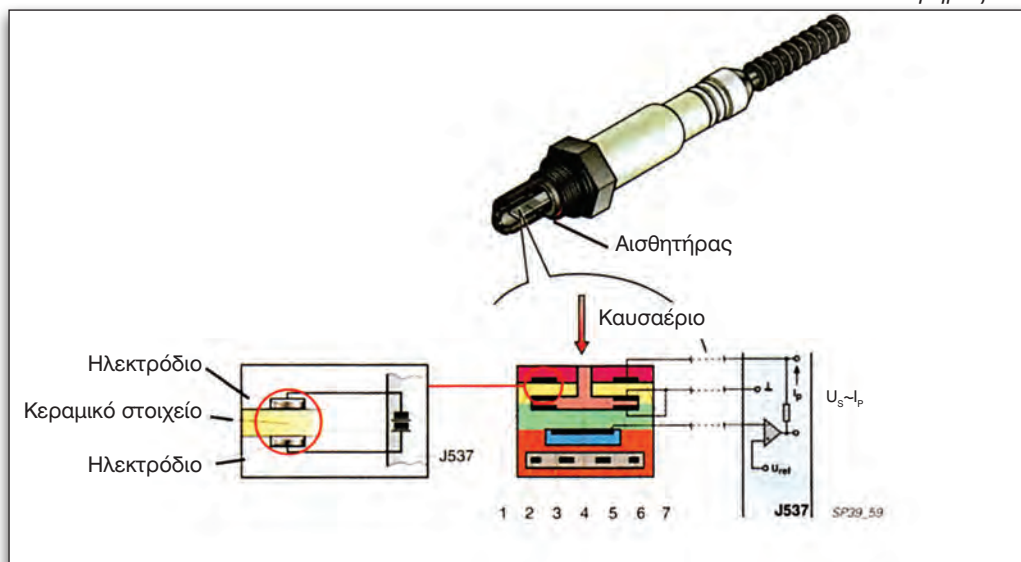
Εικόνα 4.2.13 Αισθητήρας “λ”.
