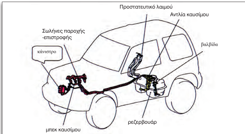
Εικόνα 3.1.6 Κύκλωμα βενζίνης
