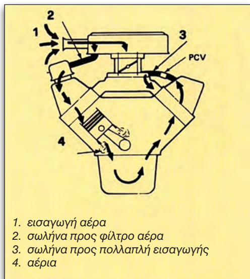
Εικόνα 4.1.14 Αερισμός στροφαλοθαλάμου
