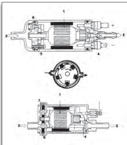
1. οπλισμός, 2. έξοδος καυσίμου, 3. είσοδος καυσίμου, 4. βαλβίδα ελέγχου, 5. δίσκος με εγχοπές, 6. ανακουφιστική βαλβίδα, 7. πλευρικό κανάλι, 8. περιφερειακή αντλία
