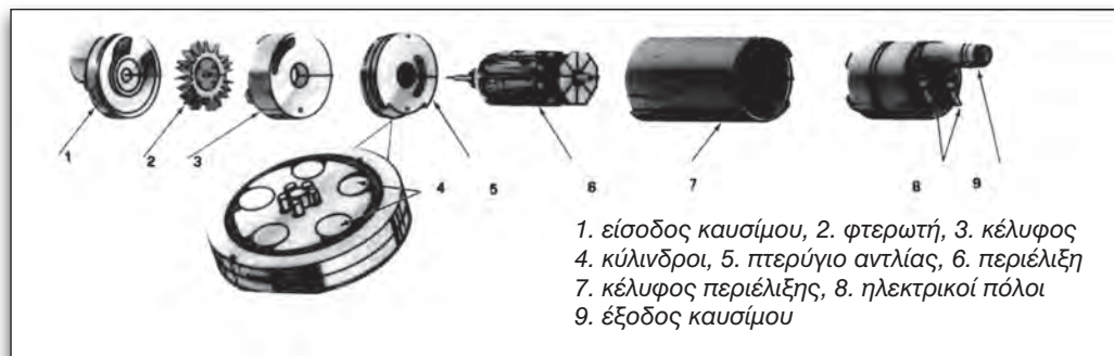
Εικόνα 3.1.12 Μέρη αντλίας καυσίμου
