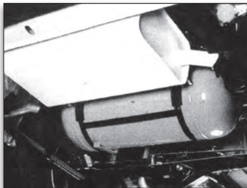
Εικόνα 7.1.3 Τοποθέτηση δοχείου αποθήκευσης υγραερίου κάτω από το δάπεδο του αυτοκινήτου
