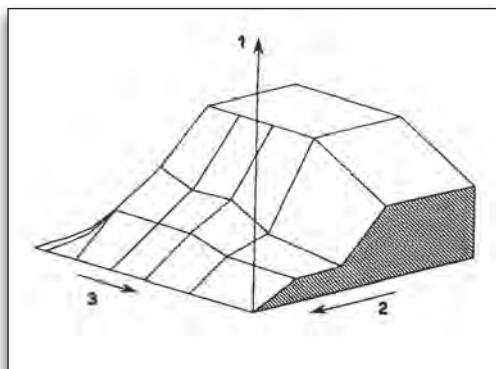
Εικόνα 3.2.9 Διορθωτικός συντελεστής κατά την περίοδο της προθέρμανσης
