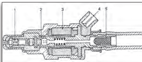
Εικόνα 3.1.16 Μπεκ σε λειτουργία
