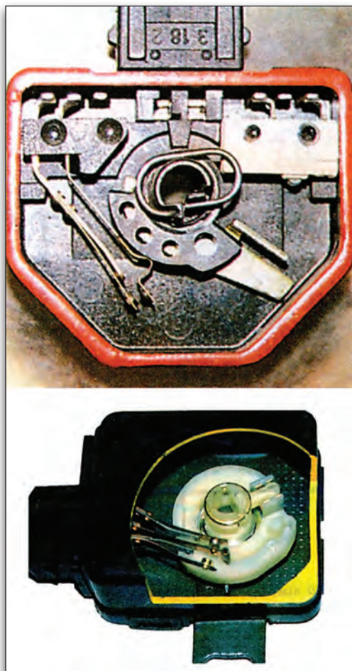
Εικόνα 3.1.36 Διακόπτης πεταλούδας
