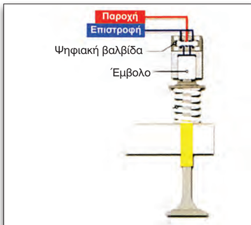
Εικόνα 2.3.11 Σύστημα υδραυλικής κίνησης βαλβίδων
