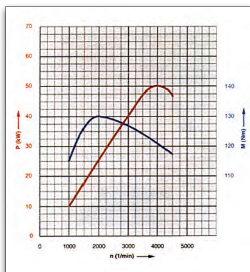
Εικόνα 8.1.1. Διάγραμμα Ισχύος - Ροπής και στροφών κινητήρα (κόκκινη καμπύλη - ισχύς, μπλε καμπύλη - ροπή)
