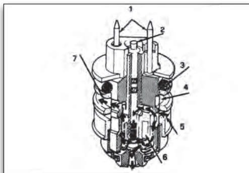
Εικόνα 3.1.18 Μπεκ κεντρικού ψεκασμού 6 οπίων γωνίας ψεκασμού 45° με σφαιρική έδραση
