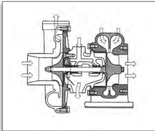
Εικόνα 2.5.4 Στροβιλοσυμπίεστής
