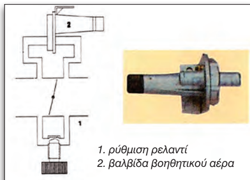
Εικόνα 3.1.39 Μπάι-πας και βαλβίδα βοηθητικού αέρα (τσοκ)
