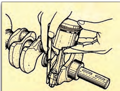
Εικόνα 2.2.9 Μέτρηση αξονικής ανοχής μεταξύ μπιέλας και στροφάλου
