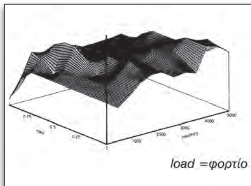
Εικόνα 3.2.11 Χάρτης διόρθωσης μείγματος
