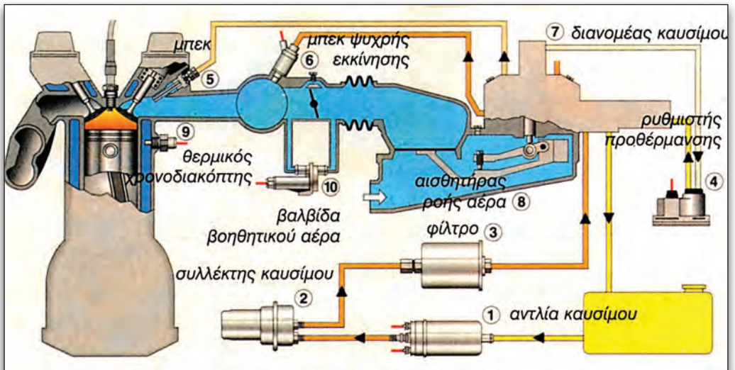
Εικόνα 3.1.44 Σύστημα K-Jetronic
