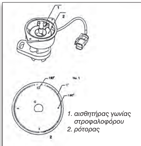
Εικόνα 3.2.16 Αισθητήρας και δίσκος με σχισμές
