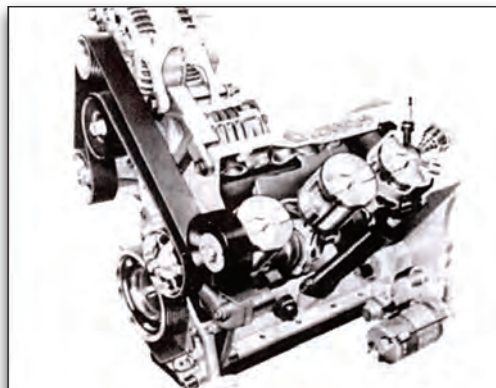
Εικόνα 1.2.8 Δίχρονος βενζινοκινητήρας
