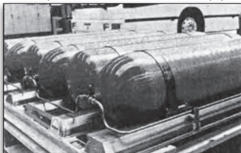
Εικόνα 7.1.9 Φιάλες αποθήκευσης φυσικού αερίου που τοποθετούνται σε λεωφορεία
