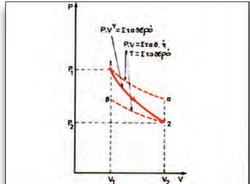
Εικόνα 1.1.4 Αδιαβατική μεταβολή
