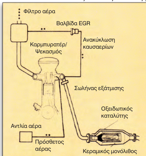
Εικόνα 4.2.2 Οξειδωτικός καταλύτης
