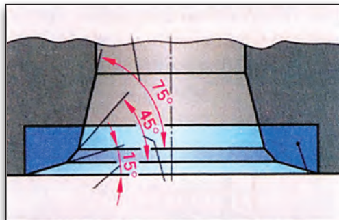
Εικόνα 2.1.5 Γωνίες λείανσης έδρας βαλβίδων
