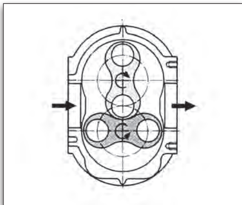
Εικόνα 2.5.2 Ελικοειδής υπερσυμπίεστής
