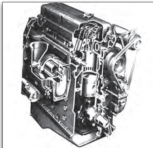
Εικόνα 1.2.13 Δίχρονες πετρελαιομηχανές
