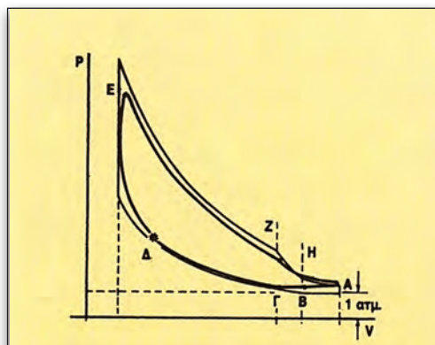
Εικόνα 1.2.10 Θεωρητική (πάνω) και πραγματική λειτουργία (κάτω) 2χρονου βενζινοκινητήρα σε διάγραμμα P-v
