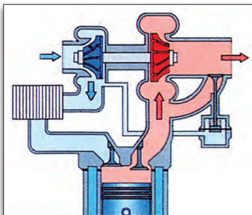
Εικόνα 2.5.5 Σχηματική διάταξη κινητήρα με στροβιλοσυμπιεστή
