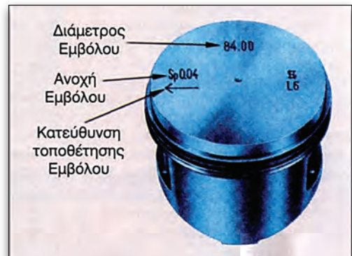
Εικόνα 2.2.6 Χαρακτηριστικά εμβόλου
