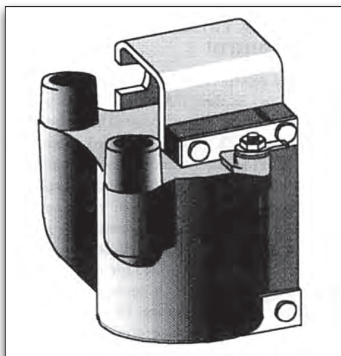
Εικόνα 3.2.22 Πολλαπλασιαστής.
