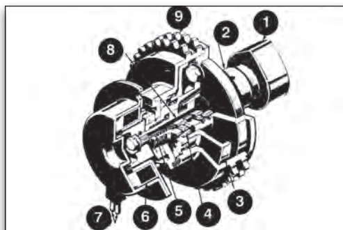
Εικόνα 2.3.8 Ηλεκτρονικά ελεγχόμενο μεταβλητό σύστημα χρονισμού. (Mercedes Benz)
