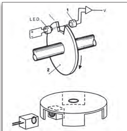
Εικόνα 3.2.5 οπτικός αισθητήρας
