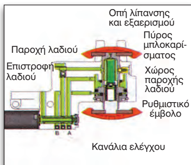
Εικόνα 2.3.7 Ρυθμιστής εκκεντροφόρου
