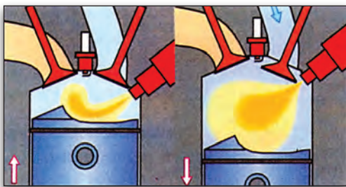
Εικόνα 3.1.4. Θάλαμος καύσης και φάσεις άμεσου ψεκασμού
