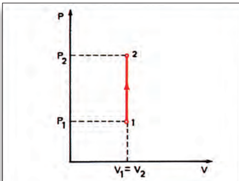
Εικόνα 1.1.3 Ισόχωρη μεταβολή
