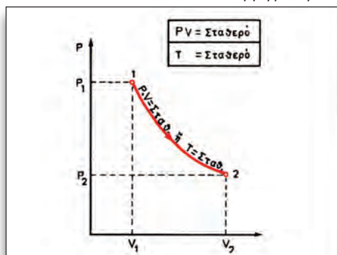
Εικόνα 1.1.1 Ισόθερμη μεταβολή
