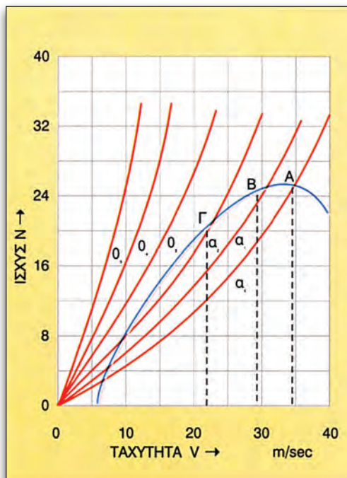
Εικόνα 8.2.11 Διάγραμμα ισχύος αντιστάσεων αυτοκινήτου κατά την κίνησή του σε οδόστρωμα με διαφορετική κλίση και ισχύος του κινητήρα.
