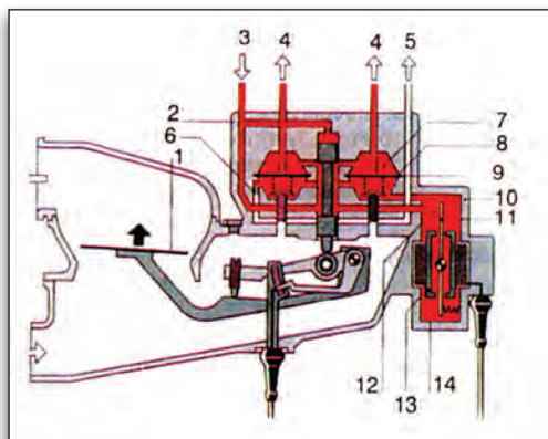
Εικόνα 3.1.49. Διανομέας με ηλεκτροϋδραυλικό ρυθμιστή
