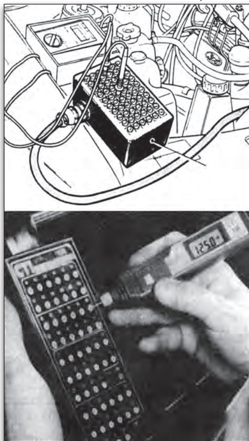
Εικόνα 5.11 Κουτιά ακροδεκτών
