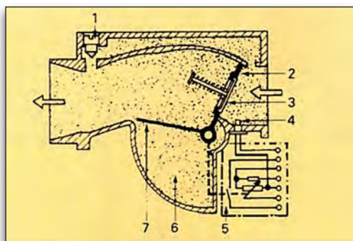
Εικόνα 3.1.27 Τομή αισθητήρα ροής
