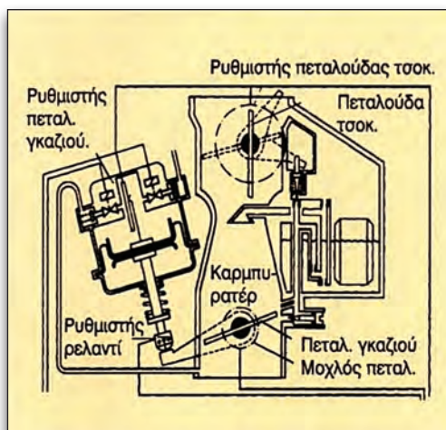
Εικόνα 4.2.11 Ηλεκτρικά ρυθμιζόμενο καρμπυρατέρ
