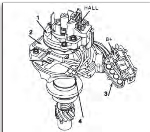
Εικόνα 3.2.6 Ανάφλεξη HEI
