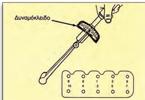
Εικόνα 2.1.4 Σειρά σύσφιγξης μπουλονιών κυλινδροκεφαλής με δυναμόκλειδο
