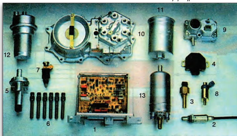
Εικόνα 3.1.45 Εξαρτήματα K-Jetronic
