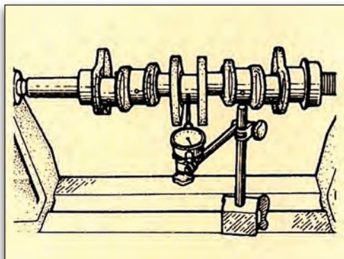
Εικόνα 2.2.8 Μέτρηση στρέβλωσης στροφαλοφόρου άξονα
