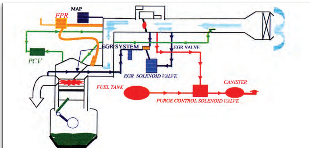
Εικόνα 4.1.1 Συνδεσμολογία και συστήματα ελέγχου ρύπων
