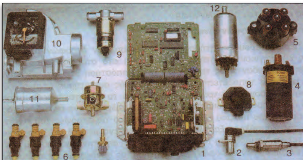
Εικόνα 3.3.4 Εξαρτήματα Motronic
