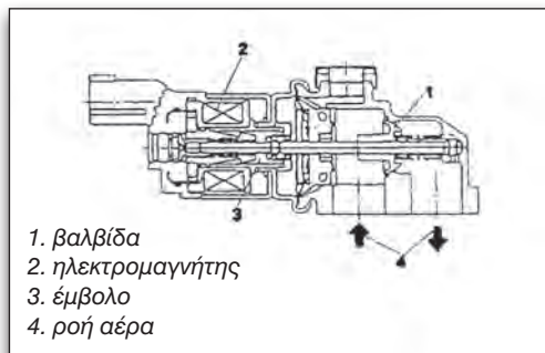
Εικόνα 3.1.40 Ηλεκτρομαγνητική βαλβίδα ρύθμισης ρελαντί
