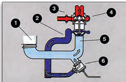
Εικόνα 2.5.11 Σύστημα με βαλβίδα ανακύκλωσης
