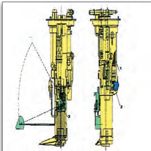
Εικόνα 3.1.9 Εμβαιπιζόμενη αντλία με φλοτέρ
