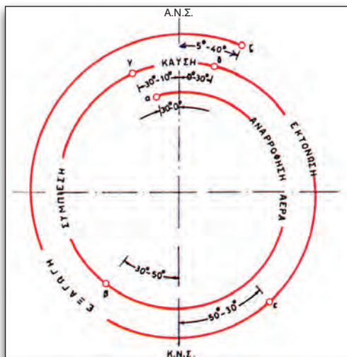
Εικόνα 1.2.7 Σπειροειδές διάγραμμα 4χρονης πετρελαιομηχανής
