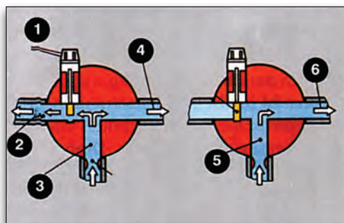
Εικόνα 2.5.8 Στιγμιαία υπερπλήρωση (Overboost)
