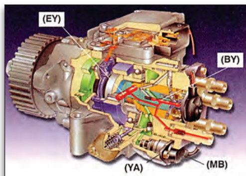
Εικόνα 6.1.5 Περιστροφική αντλία με ακτινωτή διάταξη εμβόλων.
