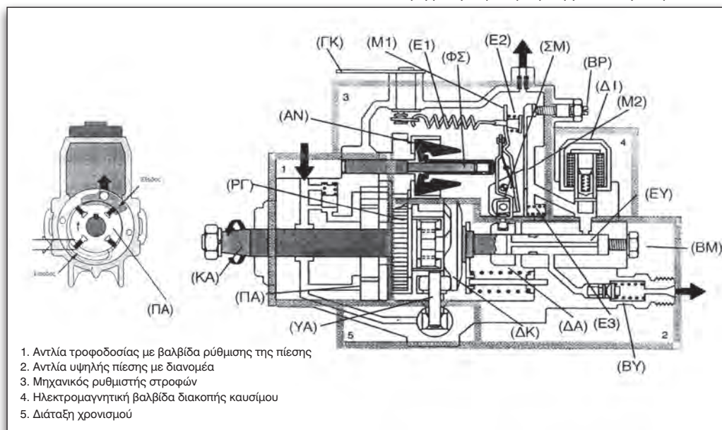
Εικόνα 6.1.2 Τομή μιας περιστροφικής αντλίας πετρελαίου.
