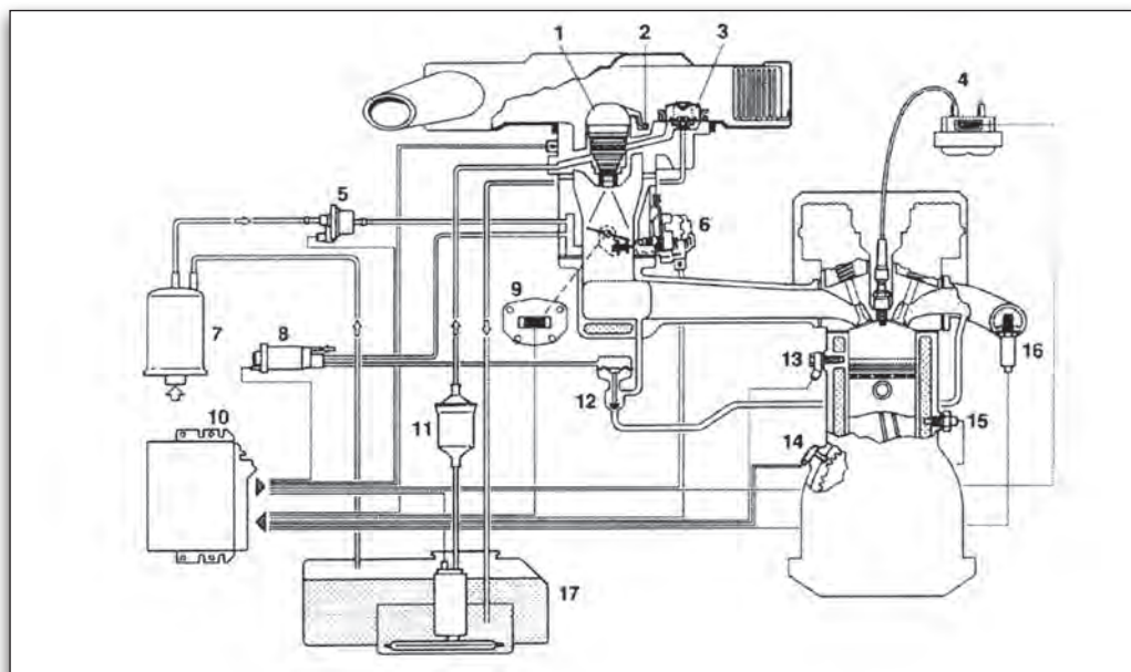
Εικόνα 3.3.7 Διάγραμμα λειτουργίας Mono - Motronic
