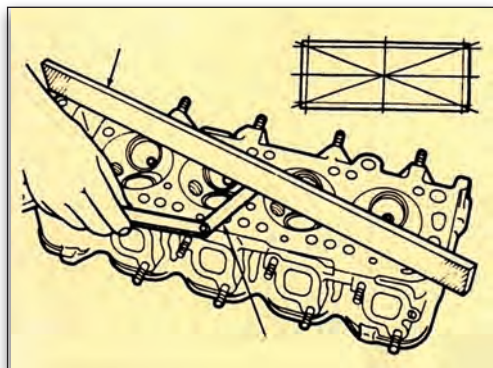
Εικόνα 2.1.3 Έλεγχος επιπεδότητας
