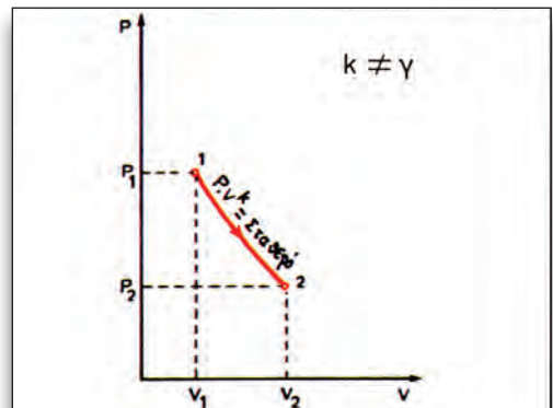
Εικόνα 1.1.5 Πολυτροπική μεταβολή
