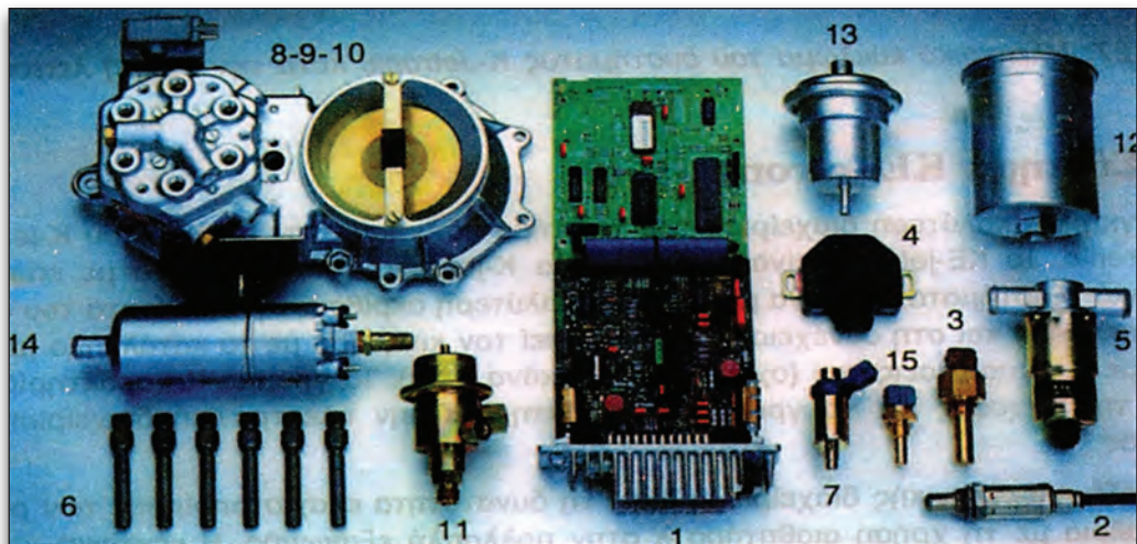
Εικόνα 3.1.47 Εξαρτήματα ΚΕ –Jetronic
