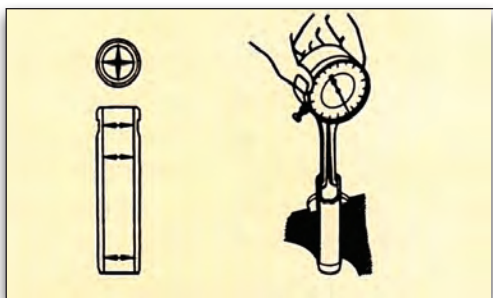
Εικόνα 2.1.8 Μέτρηση οδηγού βαλβίδας
