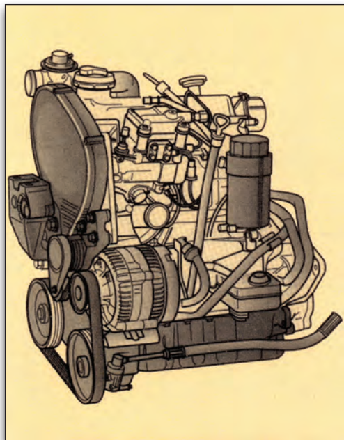
Εικόνα 6.1.1 Κινητήρας TDI
