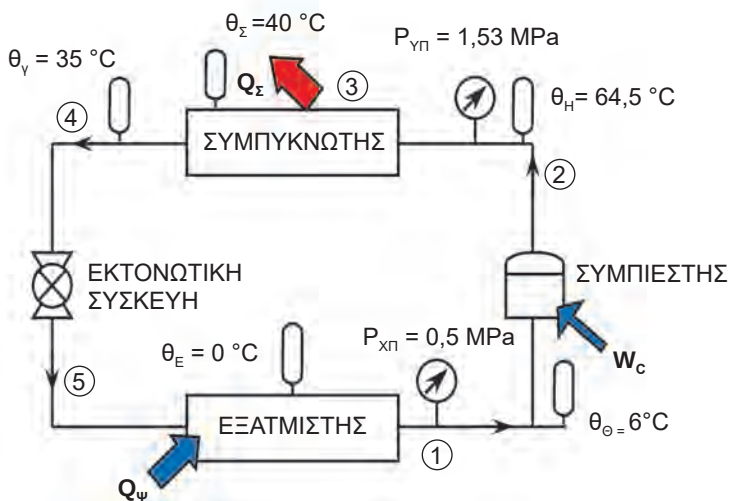
Εικόνα 1.43: Λειτουργία μιας ψυκτικής διάταξης συμπίεσης ατμών, με υπερθέρμανση και υπόψυξη. Ροή ψυκτικού ρευστού - πιέσεις - θερμοκρασίες
