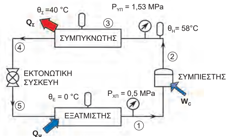
Εικόνα 1.41: Λειτουργία μιας ψυκτικής διάταξης με συμπίεση ατμών. Ροή ψυκτικού ρευστού - πιέσεις - θερμοκρασίες
