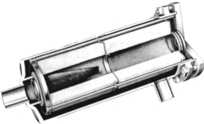
Εικόνα 7-2: Φίλτρο – Ξηραντής γραμμής υγρού
