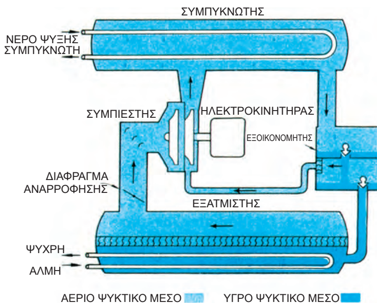
Εικόνα 2.37: Σχηματικό διάγραμμα υδρόψυκτου ψυκτικού συγκροτήματος άλμης, με ανοικτού τύπου 2-βάθμιο φυγοκεντρικό συμπιεστή
