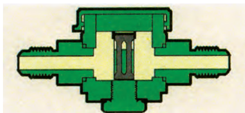
Εικόνα 7-6Β: Δείκτης ροής γραμμής υγρού – τομή
