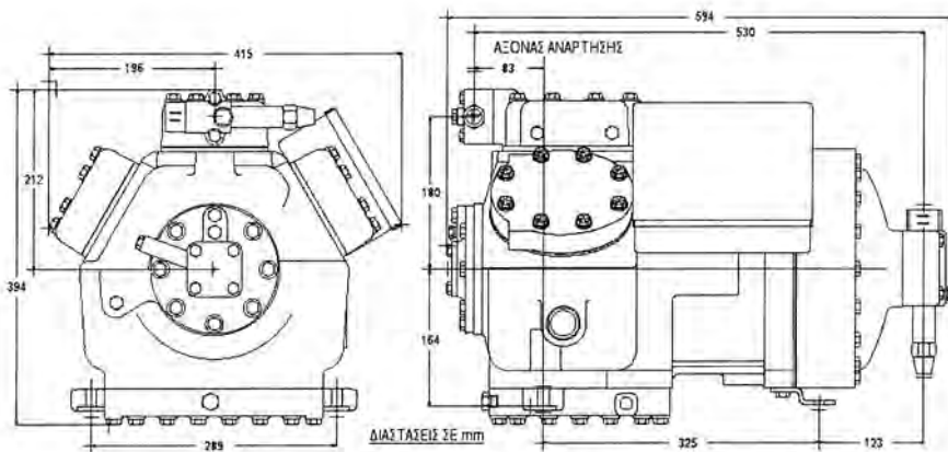
Εικόνα 2.8: Όψεις 6-κύλινδρου ημιαερμητικού παλινδρομικού συμπιεστή
