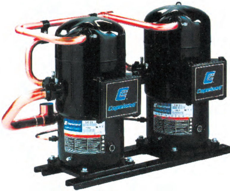
Εικόνα 2.58: Παράλληλη λειτουργία 2 ελικοειδών (Scroll) συμπιεστών με ανεξάρτητα κυκλώματα
