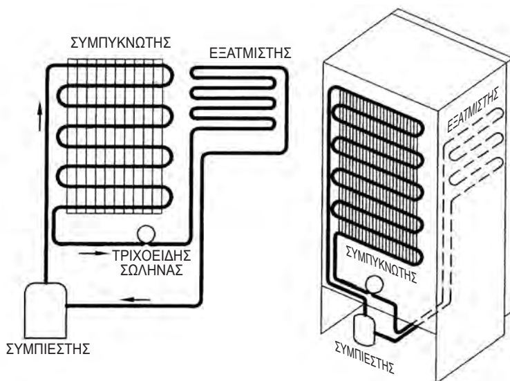
Εικόνα 3.3: Διάγραμμα οικιακού ψυγείου
