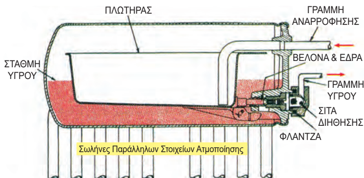
Εικόνα 5.6Α: «Εκτονωτική βαλβίδα με πλωτήρα στην πλευρά της χαμηλής πίεσης» (Low pressure float valve)
