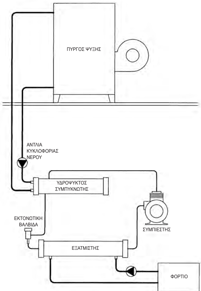
Εικόνα 4.1: Διάγραμμα υδρόψυκτης ψυκτικής εγκατάστασης
