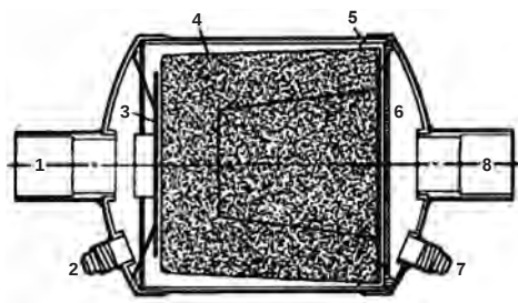
Εικόνα 7-3Α: Τομή Φίλτρου - Ξηραντή γραμμής υγρού
