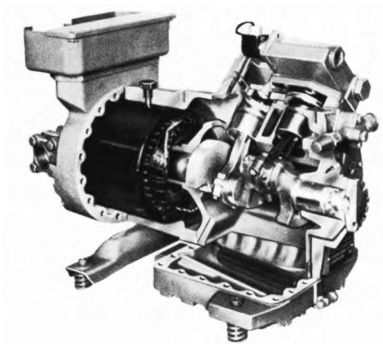
Εικόνα 2.9: Τομή ημιερμητικού παλινδρομικού συμπιεστή
