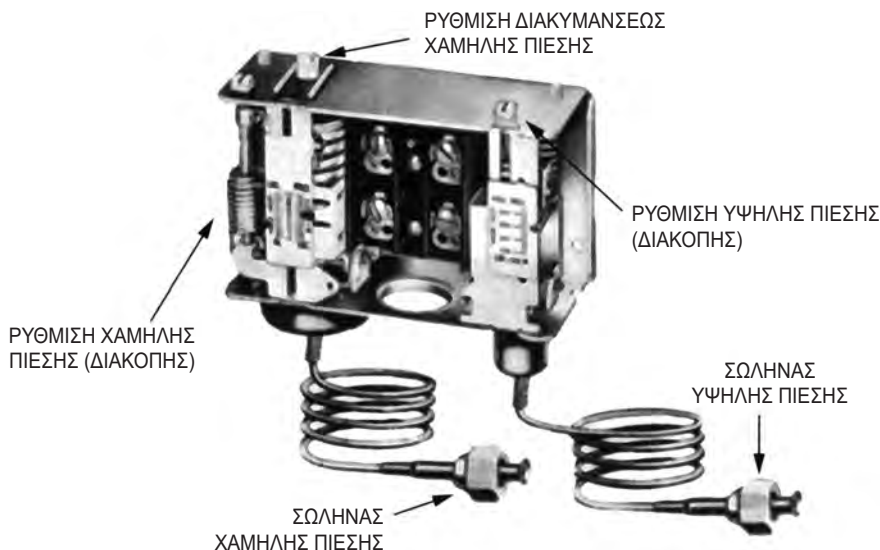
Εικόνα 7-28: Διπλός Πρεσσοστάτης με διαφορεική ρύθμιση Χαμηλής Πίεσης και προστασία Υψηλής Πίεσης
