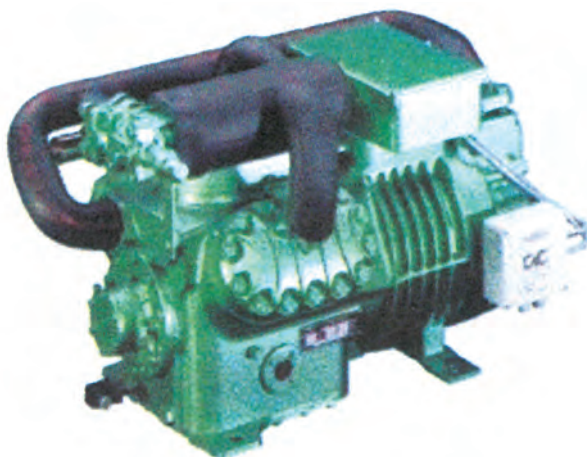
Εικόνα 2.55: Διβάθμιος ημιεργητικός παλινδρομικός συμπιεστής
