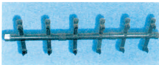
Εικόνα 4.5: Σωλήνωση διασκορπισμού νερού με ακροφύσια
