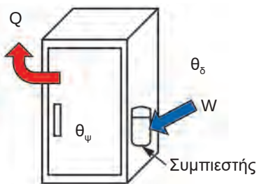
Εικόνα 1.14: Για να αφαιρέσουμε θερμότητα από το ψυγείο, είναι απαραίτητο να καταναλώσουμε ηλεκτρική ενέργεια στο συμπιεστή
