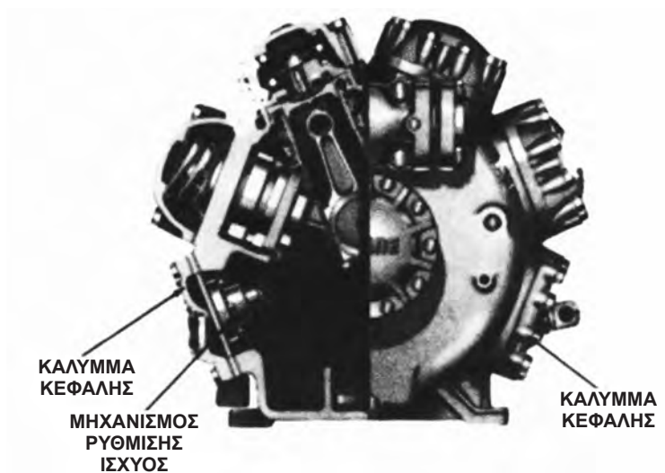
Εικόνα 2.10: Όψη και τομή 8-κύλινδρου παλινδρομικού συμπιεστή
