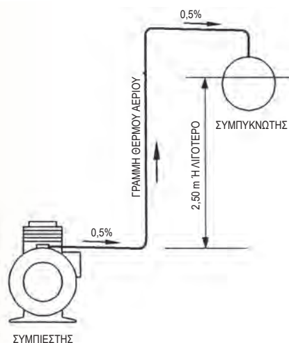
Εικόνα 9-10: Ο συμπυκνωτής υψηλότερα από το συμπιεστή με υψομετρική διαφορά μέχρι 2,50 m
