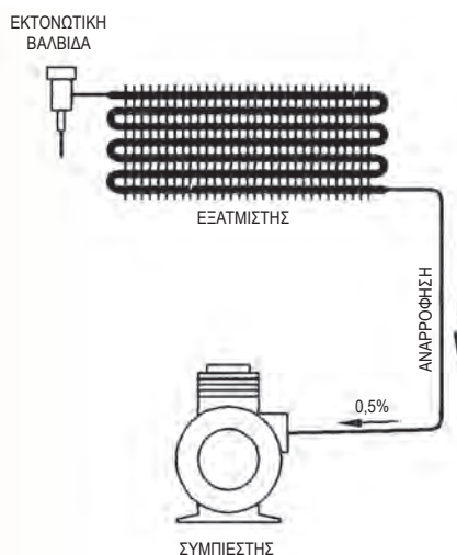
Εικόνα 9-4: Ο εξατμιστής υψηλότερα από το συμπιεστή
