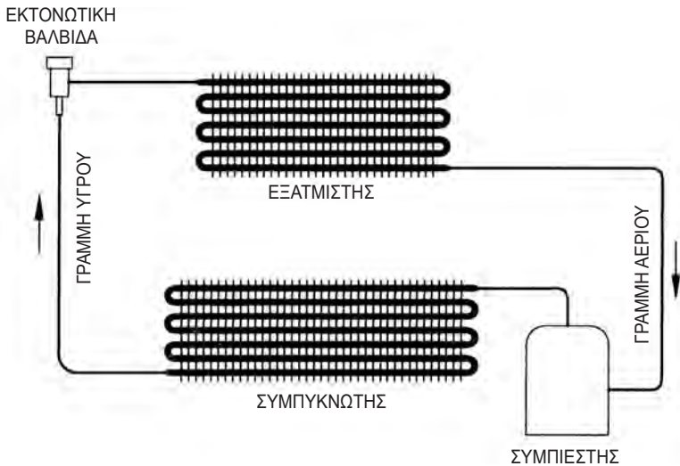
Εικόνα 3.1: Ο συμπυκνωτής μέσα στο κύκλωμα μίας ψυκτικής μηχανής
