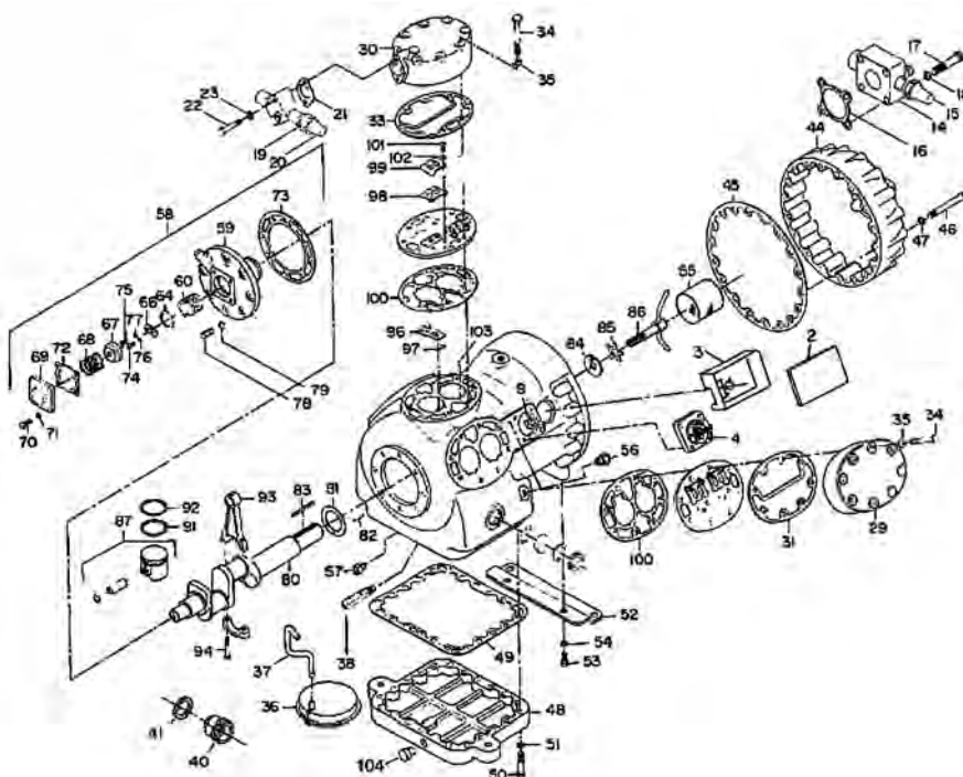
Εικόνα 2.13: Εξαρτήματα 6-κύλινδρου ημιερμητικού παλινδρομικού συμπιεστή
