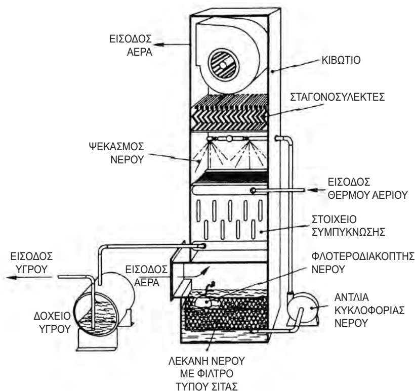
Εικόνα 3.12: Εξατμιστικός συμπυκνωτής
