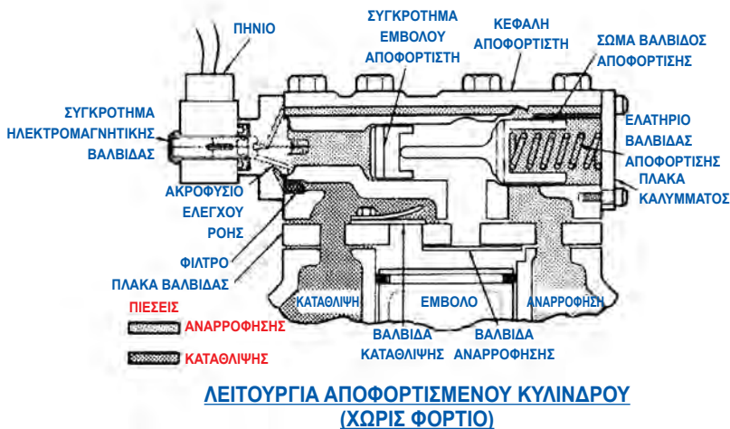
Εικόνα 2.59: Σχηματικά διαγράμματα λειτουργίας αποφορτιστή, σε παλινδρομικό συμπιεστή
