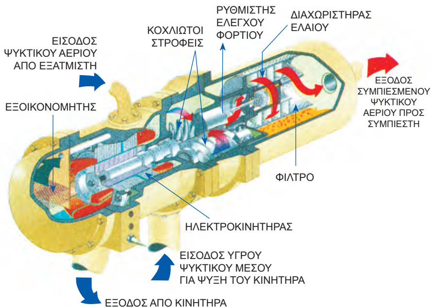
Εικόνα 2.48: Μονάδα ημι-ερμητικού κοχλιωτού συμπιεστή (screw compressor)
