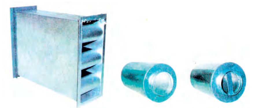
Σχήμα 8-50: Ηχοπαγίδες αεραγωγών
