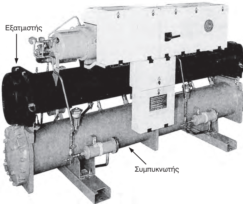
Σχήμα 7-10: Υδρόψυκτο chiller με εναλλάκτες κελύφους-σωλήνων. Οι εναλλάκτες είναι με ευθείς σωλήνες.
