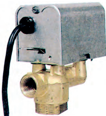
Σχήμα 8-6: Τρίοðη βάνα, κατάλληλη για τοποθέτηση σε FCU.
