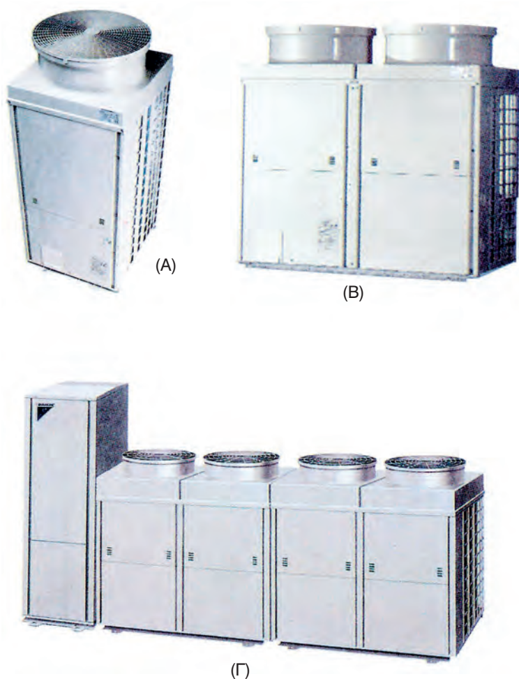
Σχήμα 6-2: Εξωτερικές μονάδες συστήματος VRV κατάλληλες για μέχρι (Α) 8 εσωτερικές κλιματιστικές μονάδες (Β) για μέχρι 16 (Γ) για μέχρι 30.
