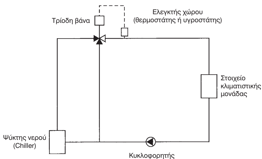
Σχήμα 10.5. Τυπική εφαρμογή τρίοδης βάνας.
