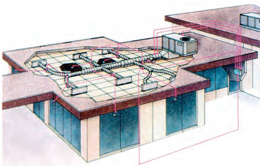
Σχήμα 9-23: Σύστημα VAV
