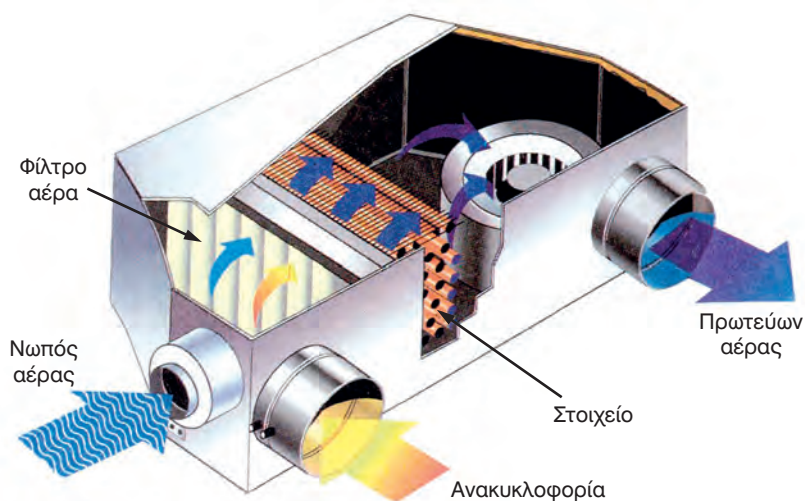
Σχήμα 9-17: Άλλος τύπος συστήματος ελέγχου της παροχής του αέρα.
