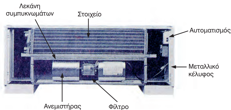
Σχήμα 8-4: Τα μέρη ενός FCU, όπως φαίνονται μονταρισμένα.
