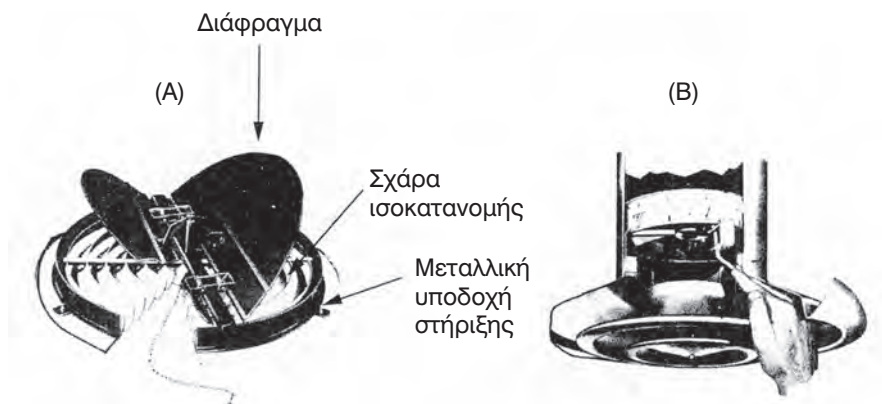
Σχήμα 5-8. Κυκλικά στόμια οροφής στα οποία φαίνονται τα εξαρτήματα από τα οποία αποτελούνται. A. Κυκλικό στόμιο οροφής με τα εξαρτήματά του. B. Ρύθμιση διαφράγματος (τάμπερ) στομίου.
