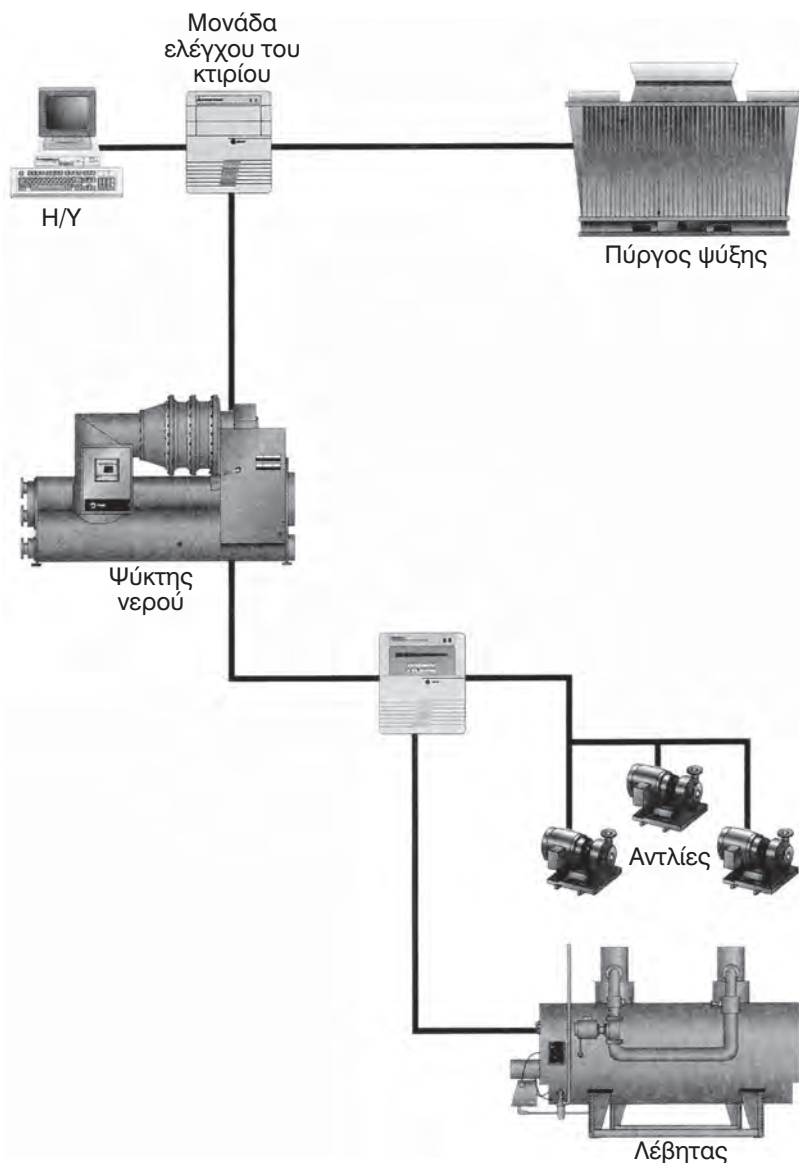
Σχήμα 10-18. Σχηματική παράσταση κεντρικού ελέγχου, μέσω H/Y, εγκατάστασης κλιματισμού.
