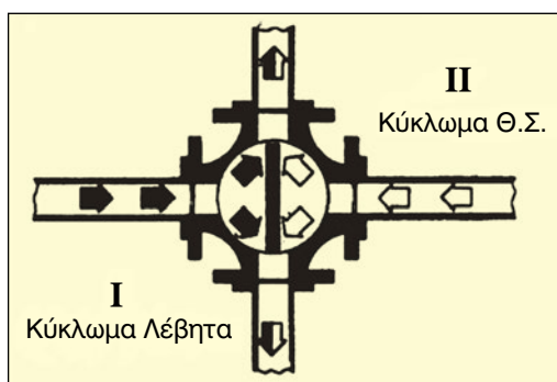
Σχήμα 3.7: Βάνα με πεταλούδα σε ενδιάμεση θέση
