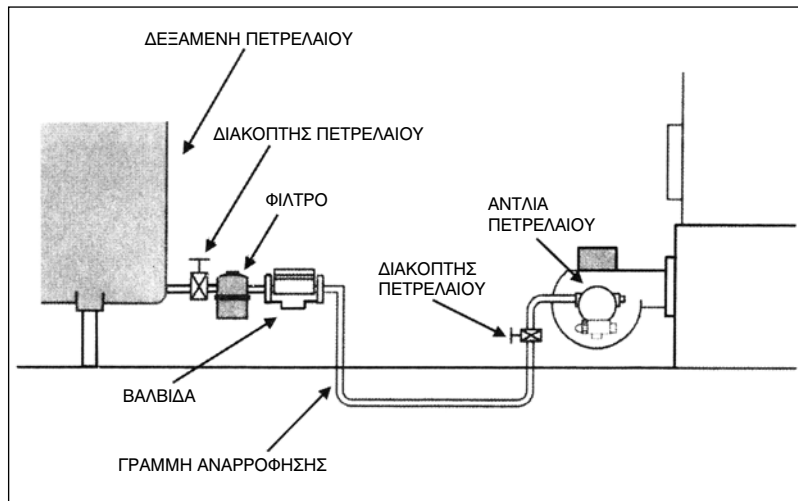
Σχήμα 1.4: Διάγραμμα σύνδεσης της δεξαμενής με τον καυστήρα
