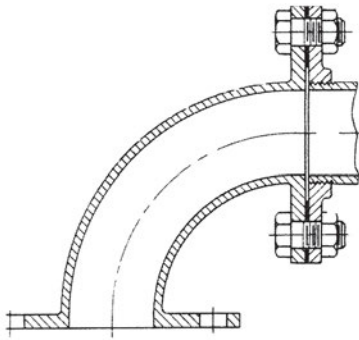
Σχήμα 3.18 (α) Σύνδεση φλαντζωτής γωνίας 90° με σωλήνα
