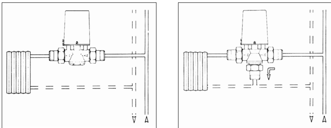
Δίοδη βαλβίδα ζώνης
