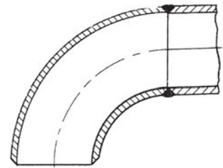
Σχήμα 3.18 (γ) Σύνδεση γωνίας 90° με σωλήνα με συγκόλληση
