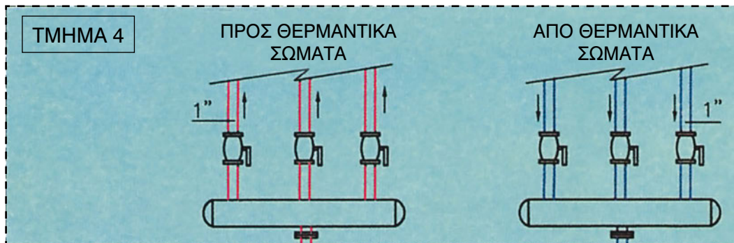
Σχήμα 3.43: Κατασκευή τμήματος σωληνώσεων διανομής Κ.Θ.-ΤΜΗΜΑ 4
