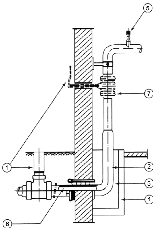
Σχήμα 1.14: Είσοδος σωλήνων διαμέσου τοίχου
