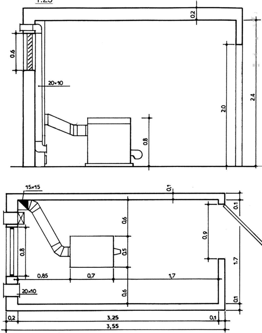
Σχήμα 3.53: Κατασκευαστικές λεπτομέρειες για την σύνδεση λέβητα με τον καπναγωγό
