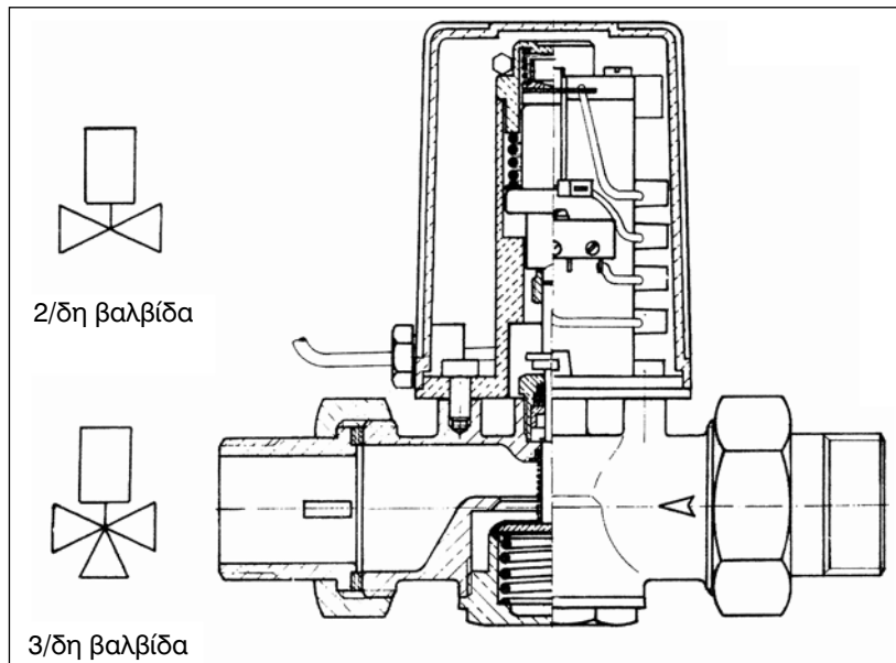
Σχήμα 5.7: Τομή βαλβίδας ζώνης
