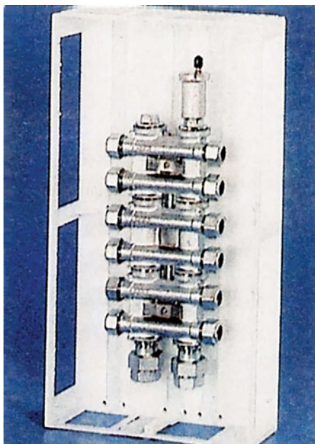
Εικόνα 4.16: Συλλέκτες μονοσωλήνιου συστήματος
