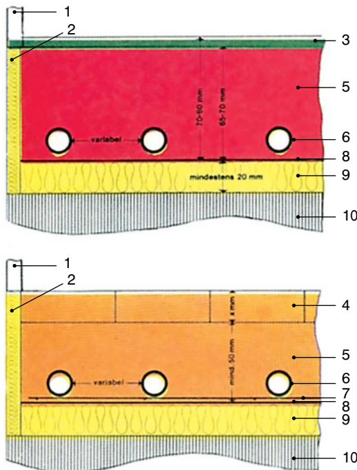
Σχήμα 4.32: Τομή δαπέδου
