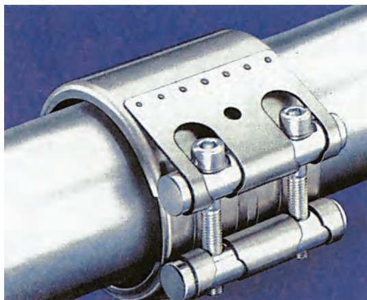
ΣΧ.8.2.2.θ Λυόμενη σύνδεση σε δίκτυο ύδρευσης.
