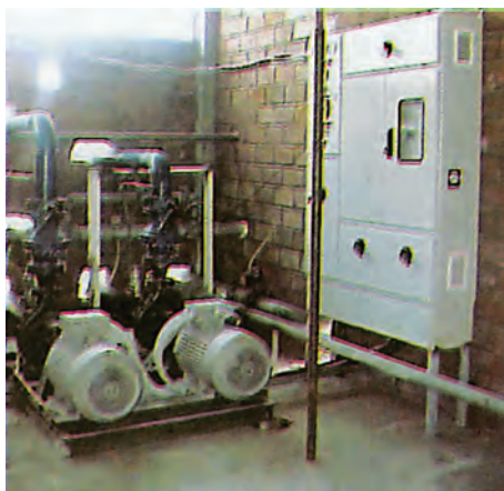
ΣΧ.9.2.3.β Βιομηχανικό αντλητικό συγκρότημα με δυο αντλίες (η μια εφεδρική) και μετατροπέα συχνότητας.
