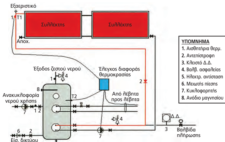
ΣΧ. 2.17.7.α Ηλιακοί Συλλέκτες και Boiler Τριπλής Ενέργειας. Το κλειστό δοχείο διαστολής (Δ.Δ.) παραλαμβάνει τις διαστολές του νερού, όταν θερμανθεί.
