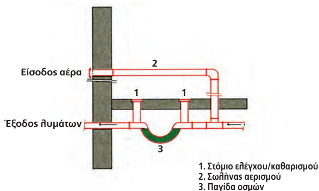
ΣΧ. 3.14.3.α Μηχανοσίφωνας
