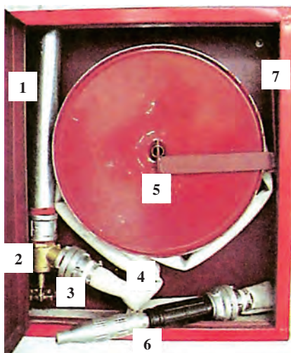
ΣΧ.10.2.1.α Εσωτερικό Πυροσβεστικής Φωλιάς.
