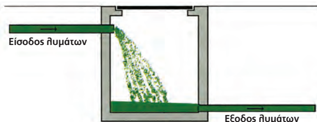
ΣΧ. 3.14.5.α Απλό φρεάτιο αποχέτευσης.
