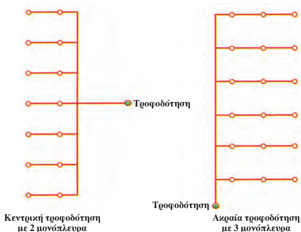
ΣΧ. 10.2.5.β Μονόπλευρη διάταξη καταιονητήρων.
