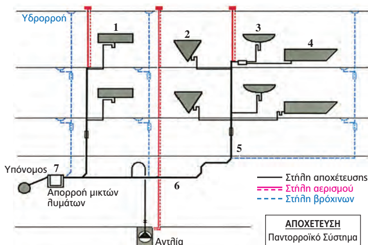
ΣΧ. 3.3.α Κατακόρυφο διάγραμμα αποχέτευσης στο παντορροϊκό σύστημα. Βασικά στοιχεία του είναι οι νεροχύτες (1), οι λεκάνες (2), οι νιπτήρες (3), οι μπανιέρες (4), οι κατακόρυφες σωληνώσεις (5), οι οριζόντιες σωληνώσεις (6) και τα φρεάτια (7).
