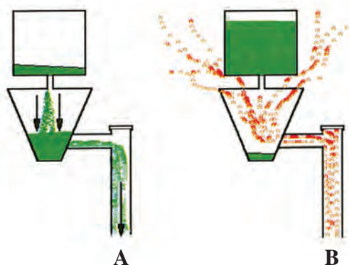
ΣΧ. 3.6.4.α Σιφωνισμός σε λεκάνη αποχέτευσης. Η απουσία του σωλήνα αερισμού έχει ως αποτέλεσμα το σιφωνισμό και το άδειασμα όλου του νερού της λεκάνης. Χωρίς οσμοπαγίδα, πλέον, τα αέρια του δικτύου αποχέτευσης μπαίνουν μέσα στις οικοδομές.
