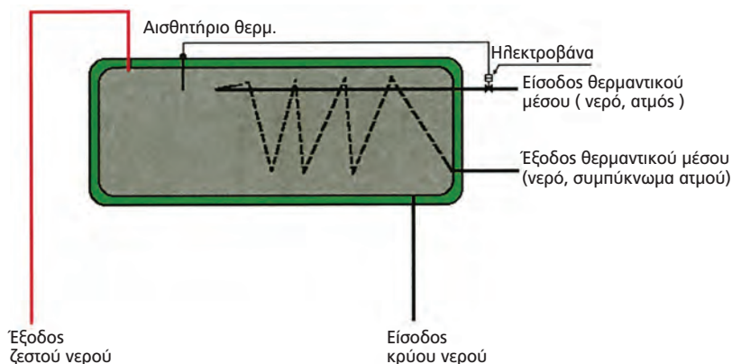
ΣΧ. 2.17.8.α Κέντρο παραγωγής ζεστού νερού.
