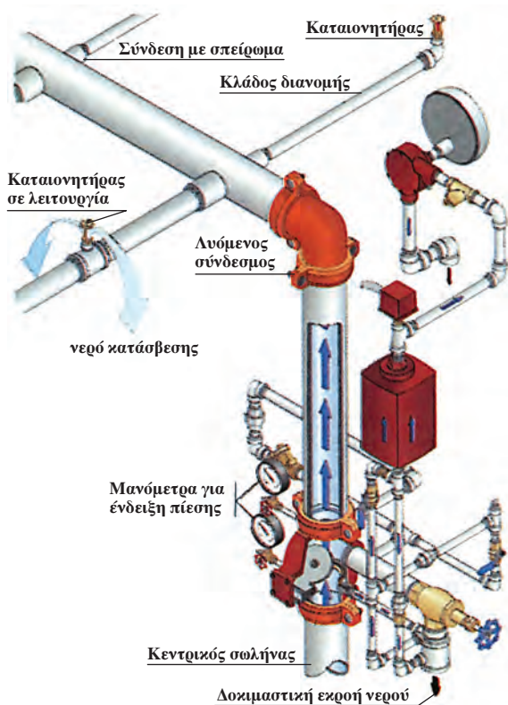
ΣΧ.10.6.α Λεπτομέρειες από κεντρικό δίκτυο πυρόσβεσης. Διακρίνονται τα βασικά στοιχεία του και οι μηχανισμοί ελέγχου της καλής λειτουργίας.
