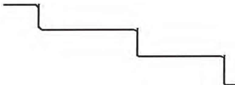
ΣΧ. 3.14.5.β Φρεάτια πτώσης στάθμης και κατακόρυφη μετατόπιση αγωγών αποχέτευσης.
