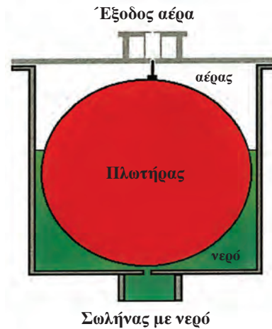
ΣΧ. 2.18.4.α Αυτόματο εξαεριστικό
