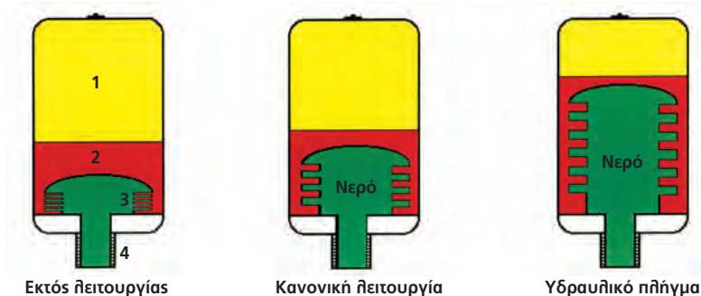
ΣΧ. 2.18.12.α Αντιπληγματικά.
