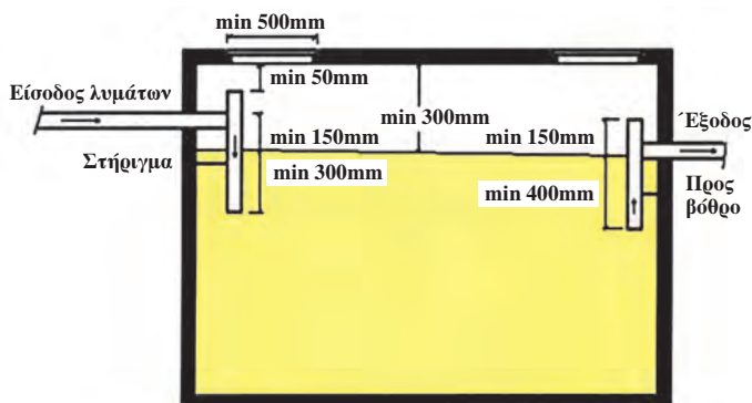
ΣΧ.5.2.1.α Μονοθάλαμος στεγανός βόθρος.
