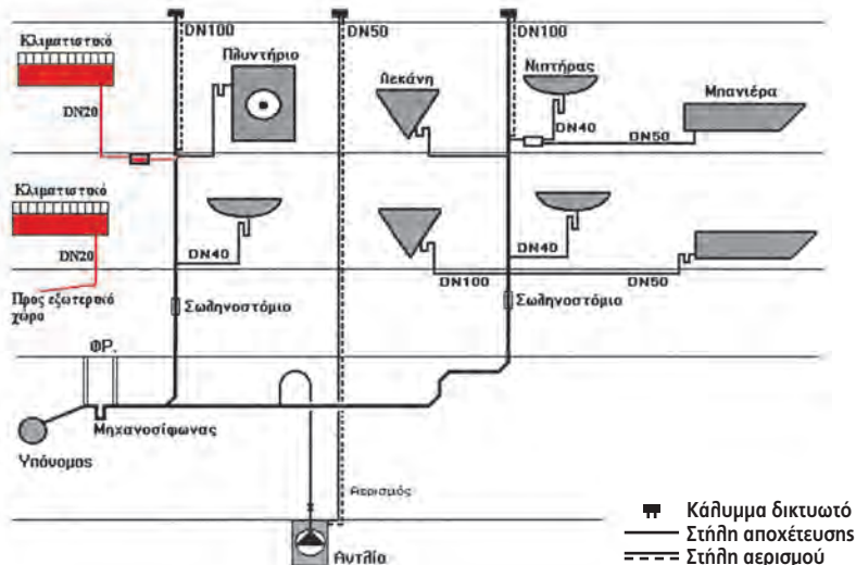
ΣΧ. 3.9.γ Κατακόρυφο σχέδιο αποχέτευσης με είδη υγιεινής και κλιματιστικά. Οι κλιματιστικές συσκευές αποχετεύονται είτε σε σιφόνια δαπέδου, που γεμίζουν συνεχώς με νερό, είτε έξω στο περιβάλλον. Δε συνδέονται ποτέ απ' ευθείας σε στήλες αποχέτευσης.
