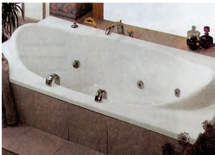
Σχ.7.3.δ Μπανιέρα με υδρομασάζ. Διακρίνονται τα στόμια εισόδου του νερού για το μασάζ. Κάτω ή δίπλα από τη μπανιέρα τοποθετείται αντλία ανακυκλοφορίας του νερού.
