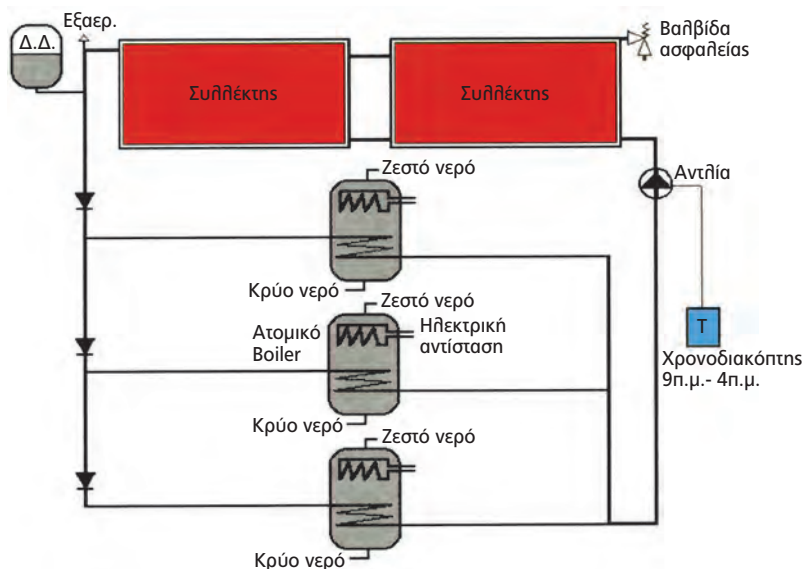
ΣΧ. 2.17.2.ζ Κεντρικοί ηλιακοί συλλέκτες ζεστού νερού χρήσης σε πολυκατοικία. Κάθε ιδιοκτησία έχει το δικό της παρασκευαστήριο.
