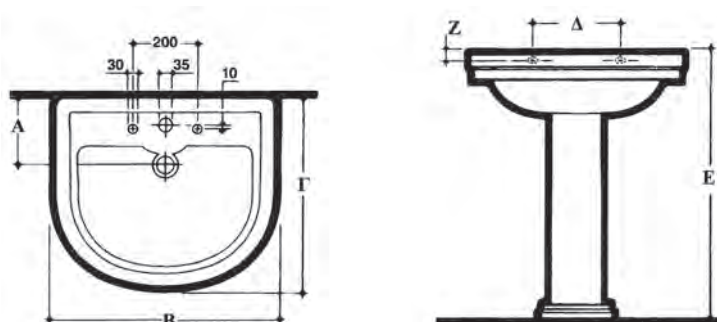
ΣΧ.7.4.α Νιπτήρας και βασικές του διαστάσεις.
