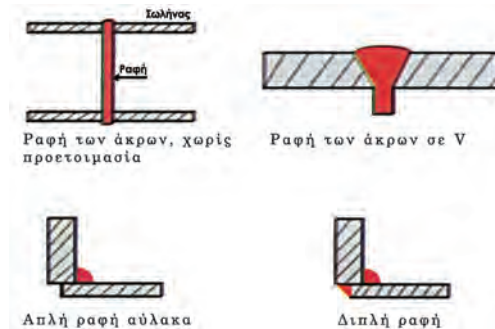
ΣΧ. 8.2.2.η Ραφές συγκολλήσεων.
