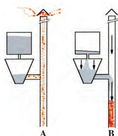
ΣΧ. 3.6.3.α Λειτουργία στήλης αποχέτευσης - αερισμού
