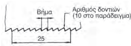
Σχήμα 4.9γ Βήμα-πυκνότητα δοντιών πριονολεπίδας
