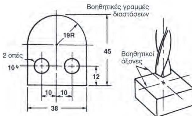
Σχήμα 4.1.1α Σχέδια χάραξης
