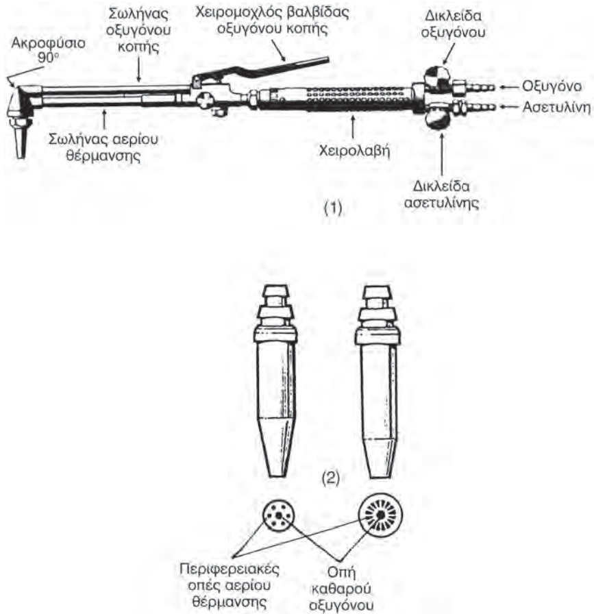
Σχήμα 8.3.12β 1) Οξυγονοκόφτης. 2) Ακροφύσια οξυγονοκόφτη.
