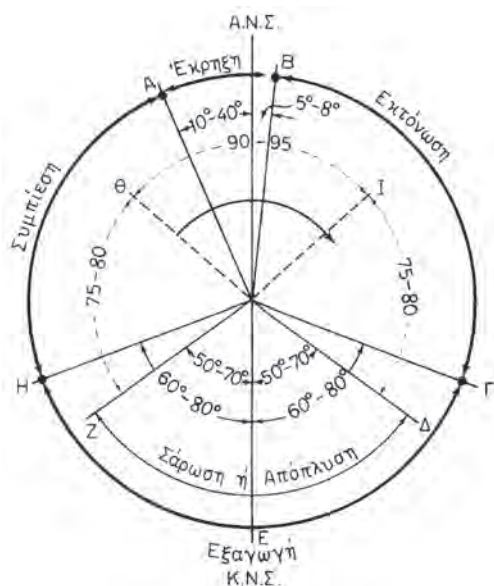
Σχήμα 14.2.1β Διάγραμμα πραγματικής λειτουργίας της δίχρονης βενζινομηχανής
