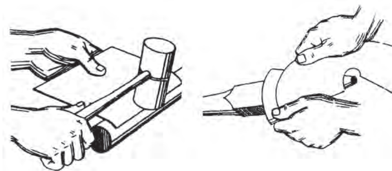
Σχήμα 6.3β Κάμψη κατά καμπύλη
