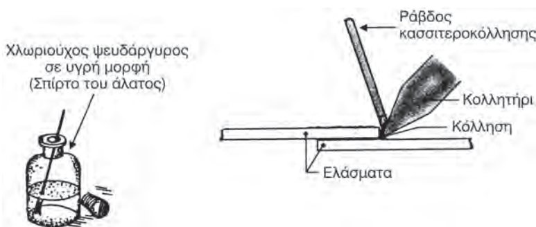
Σχήμα 8.2.2στ: Κασσιτεροσυγκόλληση ελασμάτων σε επάλληλη ένωση
