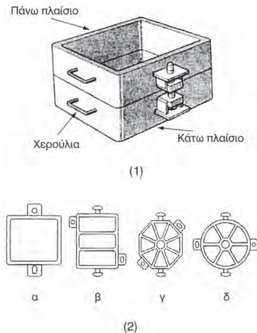
Σχήμα 10.2.1α 1. Πλαίσια χυτηρίου 2. Διάφοροι τύποι πλαισίων χυτηρίου: α) Τετράγωνος β) Ορθογωνικός γ) Πολυγωνικός δ) Κυκλικός.
