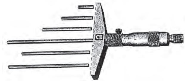
Σχήμα 3.2.5ζ Βαθύμετρο με ανταλλακτικές ράβδους
