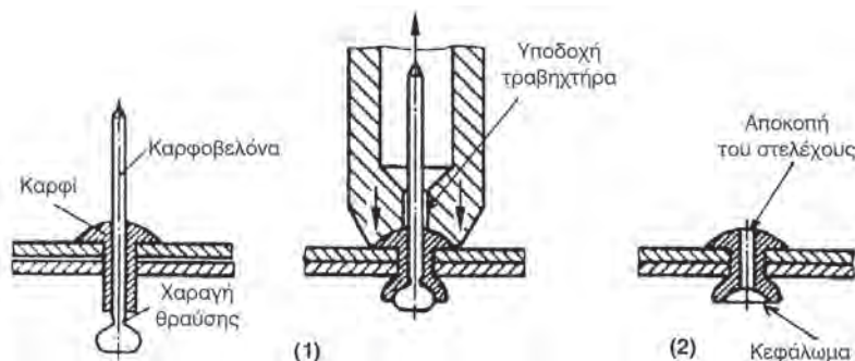
Σχήμα 7.1.2θ Καρφωτή σύνδεση με χρήση τυφλοκαρφιού και κάρφωμα με μηχανικό τραβηχτήριο (πριτσιναδόρο)
