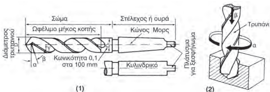
Σχήμα 4.14α -1. Τα κύρια μέρη του τρυπανιού
