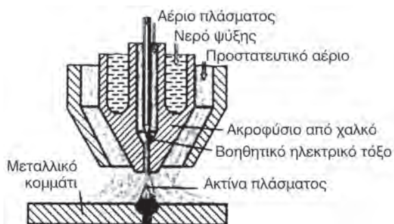
Σχήμα 8.4.10β: Ηλεκτροσυγκόλληση με μη καταναλώσιμο ηλεκτρόδιο βολφραμίου και πλάσμα (WP)
