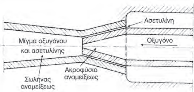
Σχήμα 8.3.7β: Τομή του καυστήρα χαμηλής πίεσεως στη θέση αναμείξεως των αερίων
