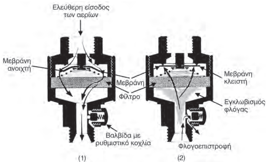
Σχήμα 8.3.6α: Βαλβίδα αντεπιστροφής σε τομή
