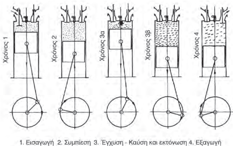
Σχήμα 14.2.3α Λειτουργία της τετράχρονης πετρελαιομηχανής
