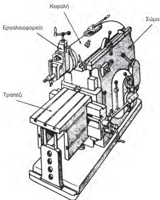
Σχήμα 13.3α Οριζόντια πλάνη (ταχυπλάνη)
