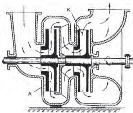
Σχήμα 16.2.1β Τομή διβάθμιου περιστροφικού αεροσυμπιεστή ακτινικής ροής A : Αναρρόφηση K : Κατάθλιψη
