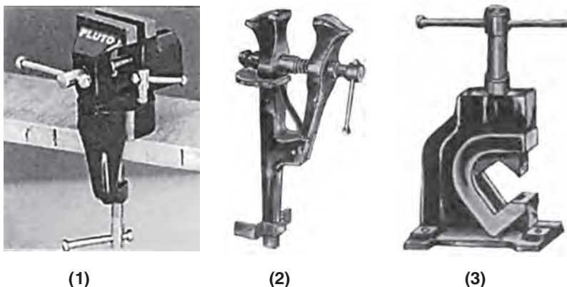
Σχήμα 4.2.2β -1. Μέγγενη εφαρμοστή -2. Μέγγενη σιδηρουργού, -3. Σωληνομέγγενη
