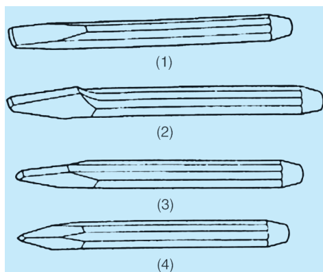
Σχήμα 4.8β -1. Πλατύ κοπίδι -2. Σταυρωτό κοπίδι -3. Μισοστρόγγυλο κοπίδι -4. Κοπίδι νύχι
