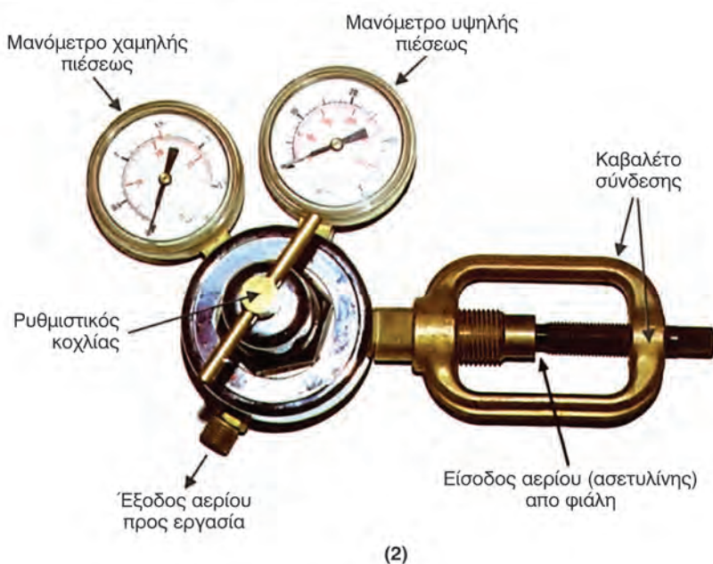
Σχήμα 8.3.4β: 1) Μανομετρικός εκτονωτής οξυγόνου. Σύνδεση στη φιάλη με τη βοήθεια μαστού. 2) Μανομετρικός εκτονωτής ασετυλίνης. Σύνδεση στη φιάλη με τη βοήθεια καβαλέτου.
