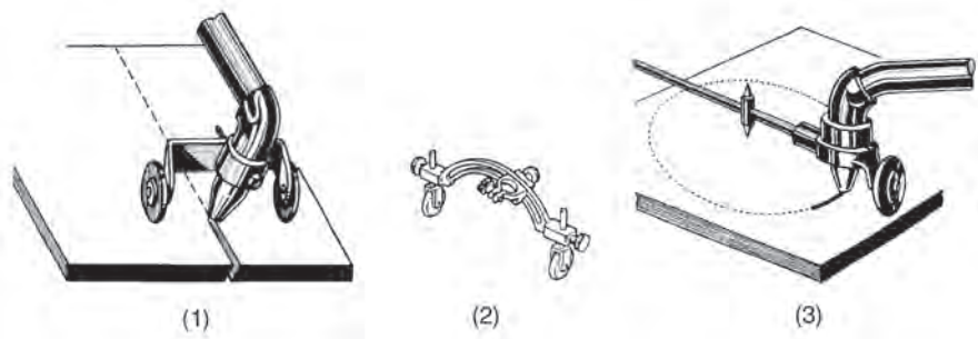
Σχήμα 8.3.12γ: 1) Ιδιοσυσσκευή με οδηγητήριους τροχούς για ευθεία οξυγονοκοπή. 2) Ιδιοσυσσκευή για οξυγονοκοπή υπό γωνία. 3) Ιδιοσυσσκευή για οξυγονοκοπή κύκλων (διαβήτη οξυγονοκοπής).
