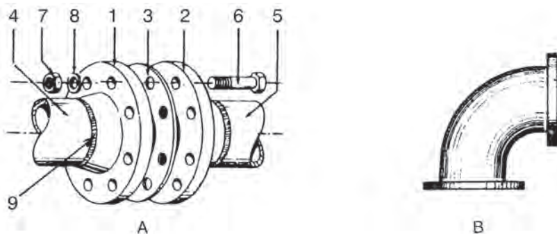
Σχήμα 9.2.1 α Α) Σύνδεση σωλήνων με φλάντζες: 1,2-Φλάντζες, 3-Παρέμβυσμα, 4,5-Σωλήνες, 6-Κοχλίας, 7-Περιοχήλιο, 8-Ροδέλλα ασφαλείας, 9-Ραφή συγκόλλησης Β) Φλαντζωτό εξάρτημα (γωνία).
