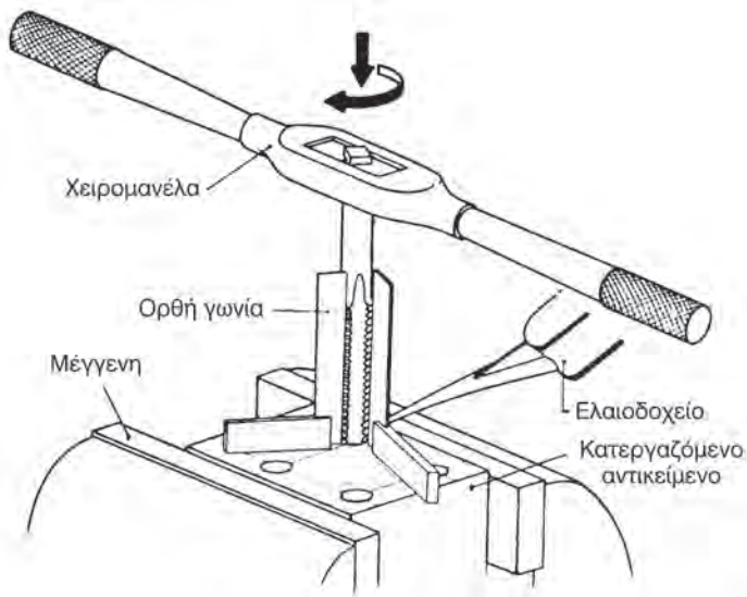
Σχήμα 4.16γ Χρήση σπειροτόμου - Έλεγχος καθετότητας με ορθή γωνιά
