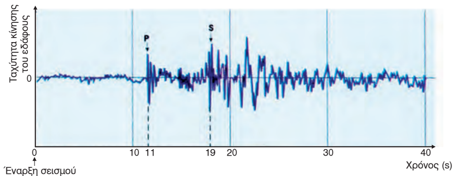
Εικόνα 5.5 Σεισμογράφημα που δείχνει το χρόνο πρώτης άφιξης των P και S κυμάτων.
