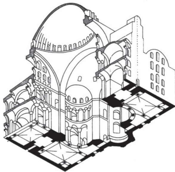
Εικ. 17. Αγία Σοφία, αξονομετρικό σχέδιο.
