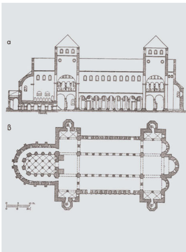
Εικ. 5. Ο ρομανικός ναός του Αγίου Μιχαήλ (1001-1033), Γερμανία, Χίλντεσάιμ (Hildesheim): α) τομή, β) κάτοψη.
