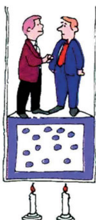
ΣΧΗΜΑ 4.6 Εικονική παρουσίαση του νόμου του Gay-Lussac. Η πίεση ενός αερίου είναι ανάλογος της απόλυτης θερμοκρασίας (με n, V σταθερά).
