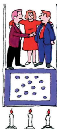
ΣΧΗΜΑ 4.6 Εικονική παρουσίαση του νόμου του Gay-Lussac. Η πίεση ενός αερίου είναι ανάλογος της απόλυτης θερμοκρασίας (με n, V σταθερά).
