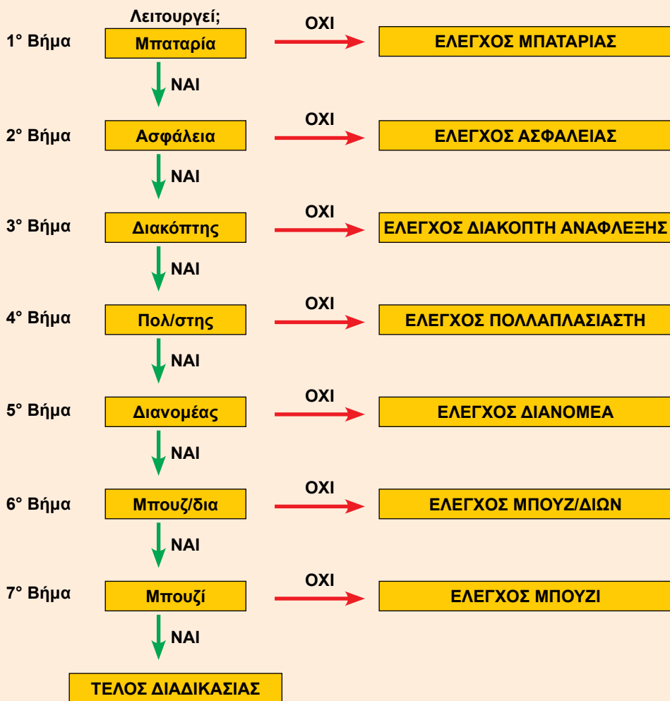
Σχήμα. 1.3: Διάγραμμα ροής εντοπισμού βλάβης.
