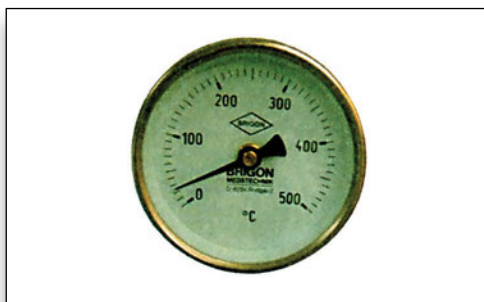
Σχήμα 2.17: Διμεταλλικό θερμομέτρο.
