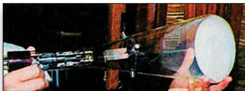
Σχήμα 2.24: Πειραματικός σωλήνας Braun.
