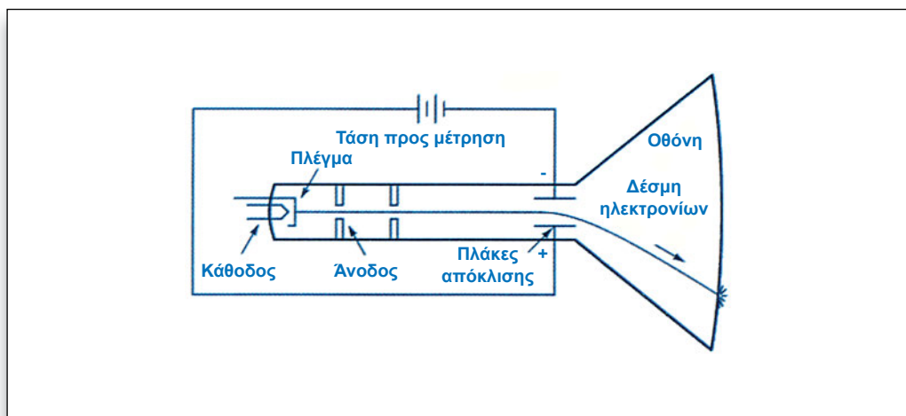
Σχήμα 2.25: Δομή και λειτουργία του καθοδικού παλμογράφου.
